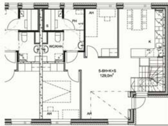
2. KERROS
