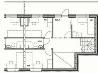
3. KERROS
