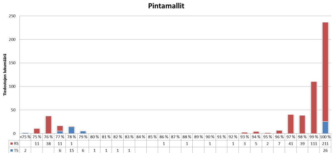
Kuva 32. Pintamallien laatu viiteaineistossa hankevaiheittain
