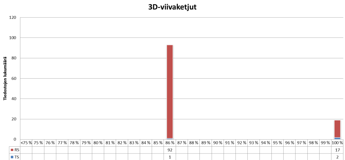
Kuva 31. 3D-viivojen laatu viiteaineistossa hankevaiheittain
