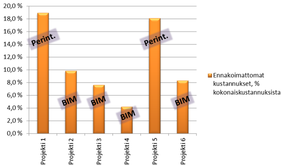
Kuva 5. Mallinnuksen kautta saavutettuja hyötyjä Norjan väylähankkeissa
