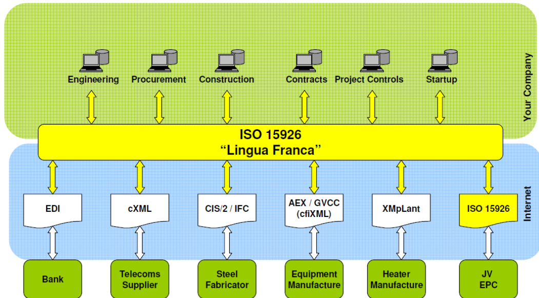
Kuva 15. ISO 15926 yhteisenä kielenä prosessiteollisuuden laitoksen elinkaareissa (Paap 2010)
