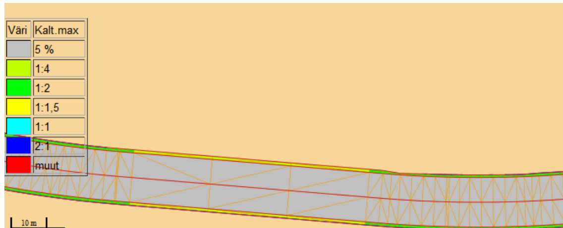
Kuva 26. Rakennussuunnitelmavaiheen aineistoa, jossa kolmiointi on osittain harvaa
