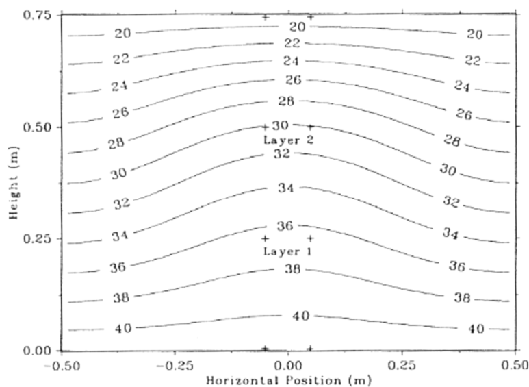
Kuva 3.4. Näytteen keskilinjän tasosta havaitut isotermit. Isotermien välinen etäisyys on alaosassa selvästi suurempi verrattuna yläosaan. (Goering et al. 2000)
