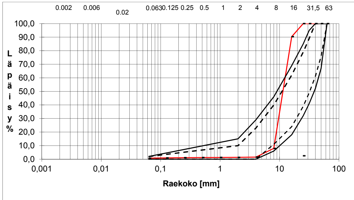
Kuva 4.22. Testattavan 5/16 mm kalliomurskeen raekokojakauma. Kuvassa mustalla piirretyt yhtenäiset viivat ovat yksittäisen rakeisuustuloksen vaihteluvälit. 90 % tuloksista tulee sijaita katkoviivoilla piirretyllä alueella.
