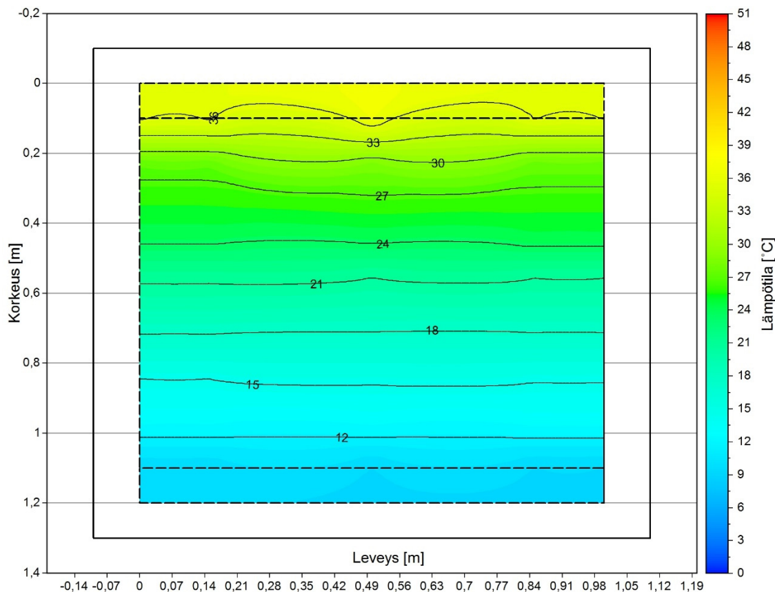
Kuva 5.1. Poikkileikkaus raideseppelinäytteen lämpötilajakaumasta ylälämmitystilanteessa lämpötilaerolla 27 °C. Lämpötilamuutos on lineaarinen ja isotermit ovat vaakasuorassa.
