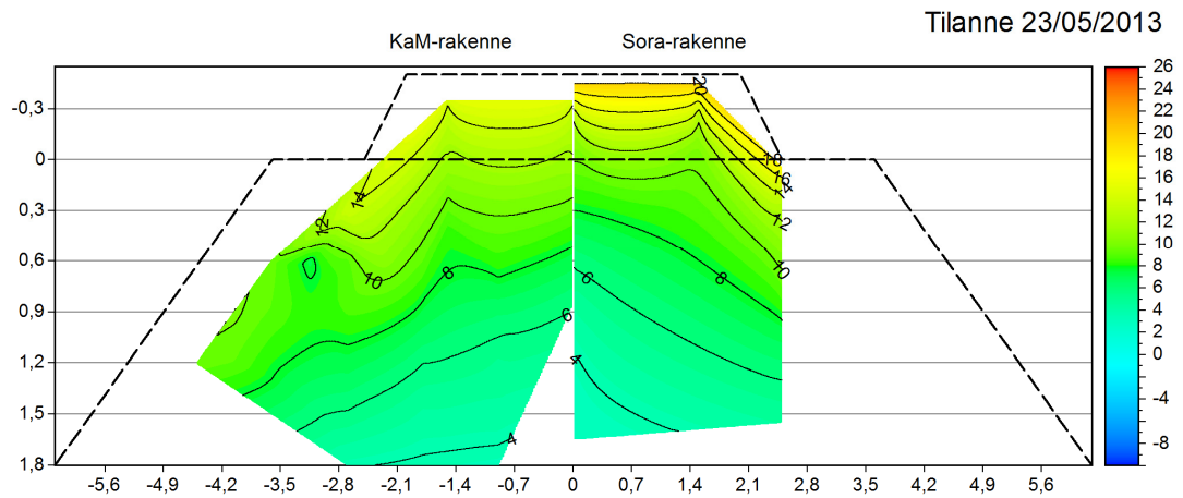
Kuva 6.12. Lämpötilat penkereissä 23.5.2013. Kalliomurske lämpenee keväällä nopeammin.
