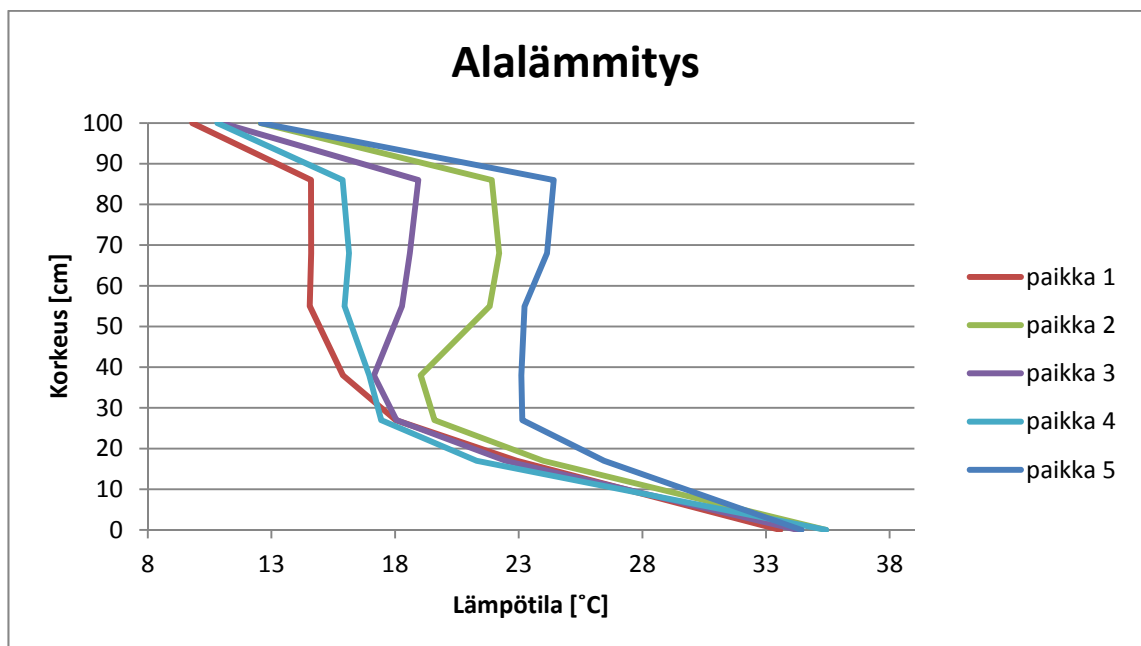
Kuva 5.9. Lämpötilat korkeuden suhteen konvektiotilanteessa. Kostealla raideseipelillä konvektio oli voimakasta ja samalla tasolla lämpötilat poikkeavat merkittävästi toisistaan. Paikka 3 on näytteen keskeltä ja muut ovat nurkkapisteitä.
