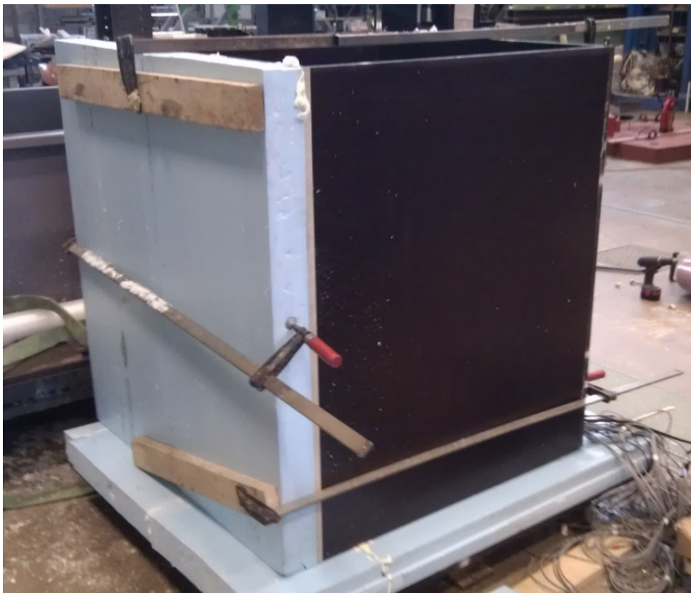
Kuva 4.5. Näytetilan eristäminen 100 mm XPS-eristeellä. Eristeet on liimattu kiinni filmivanerin pintaan ja raot on tukittu uretaanivaahdolla.
