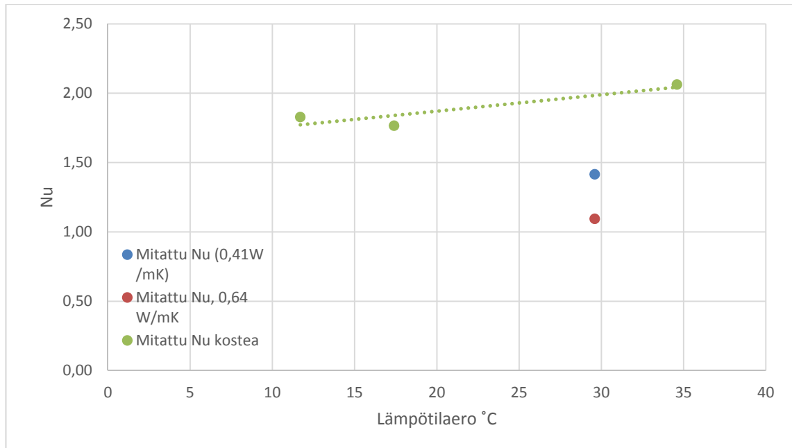
Kuva 5.29. EV-materiaalin Nusseltin luvut. Kuvassa on piirretty kuivan tilanteen Nu käyttäen kahta eri lämmönjohtavuutta. Sinisessä pisteessä on käytetty lämmönjohtavuutta 0,41 W/mK ja konvektiotilanteessa mitattua 0,58. Punaisessa pisteessä on käytetty lämmönjohtavuutta 0,64 W/mK ja konvektiotilanteessa 0,7 W/mK sisäistä lämmönjohtavuutta.
