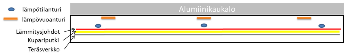
Kuva 4.18. Alalaatan poikkileikkaus. Ylälaatta on peilikuva alalaatasta, ilman lämpövuantureita. Myös alumiinikaukalon tilalla on pelkkä alumiinilevy.
