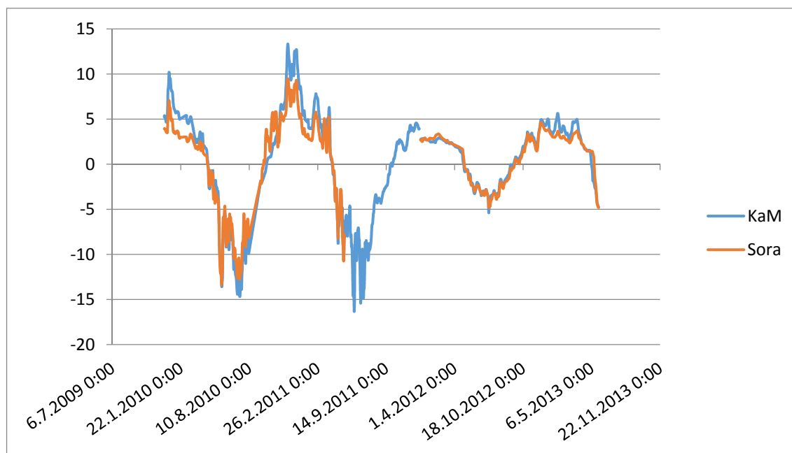
Kuva 6.17. Lämpötilaero antureiden T40 ja T7 välillä vuoteen 2011 saakka ja sen jälkeen kalliomurskerakenteessa T34 ja Tu9 ja sorarakenteessa T17 ja T5 välillä. Syksyllä 2009 sorarakenteen anturit rikkoutuivat rakennustöiden takia. Lämpötilaerot eivät ole vanhan ja uuden anturoinnin välillä suoraan verrattavissa, sillä syvyydet ovat erilaiset.
