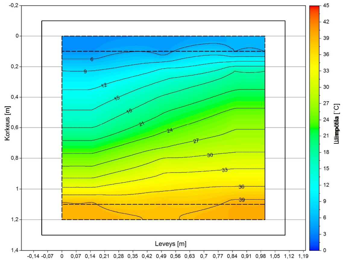
Kuva 5.16. Kostean EV-näytteen konvektiotilanne 35^{\circ}\text{C} lämpötilaerolla. Lämpö selvästi nousee toista reunaa ylös. Taitteet reunojen lähellä johtuvat approksimaatiosta.
