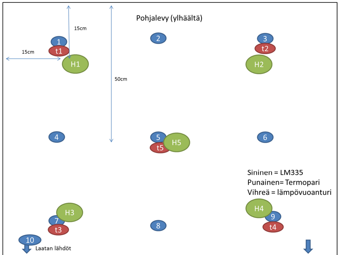
Kuva 4.17. Alalaatan antureiden sijoittelu. Ylälaatta on muuten samanlainen, mutta lämpövuanturit puuttuvat.
