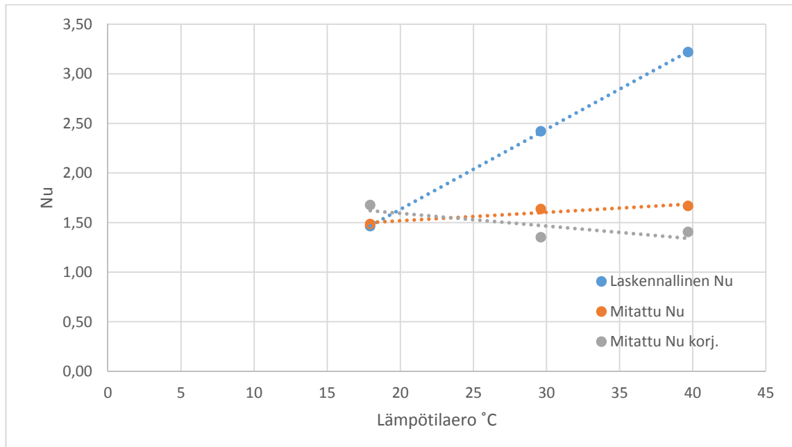
Kuva 5.26. 5/16 mm kalliomurskeelle piirretyt kuvaajat siten, että laskennassa on käytetty huomattavasti suurempaa sisäistä läpäisevyyttä 3,5 \cdot 10^{-7} \text{ m}^2 . Nu on laskettu käyttäen lämmönjohtavuutta 0,37 \text{ W/mK} .
