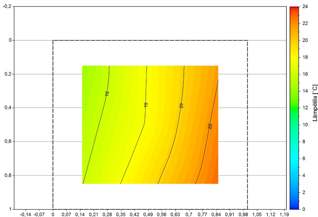
Kuva 5.3. Kostean raideseppelin lämpötilajakauma ylhäältä päin katsottuna noin 0,5 m syvyydeltä alalämmitystilanteessa. Samassa kerroksessa on suuret lämpötilavaihtelut.
