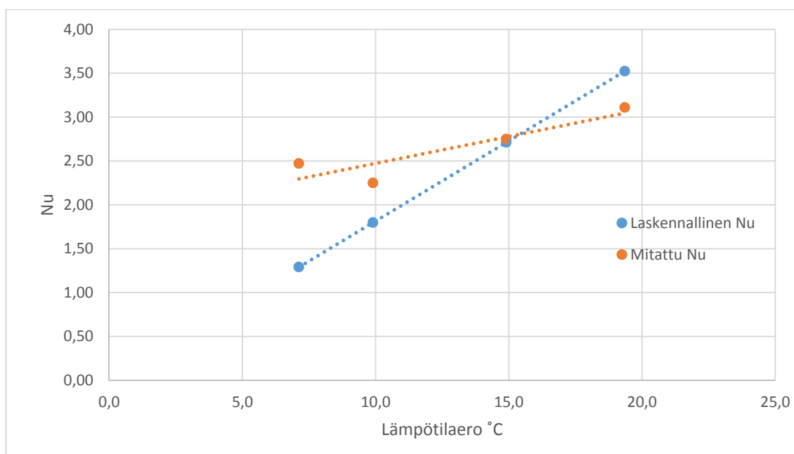
Kuva 5.22. Mitattu ja laskettu Nusseltin luku kuivalla raidesepelillä. Laskennassa on käytetty korjaamatonta lämmönjohtavuutta. Kuvassa on käytetty suoraan mitattua lämmönjohtavuutta 0,36 W/mK.
