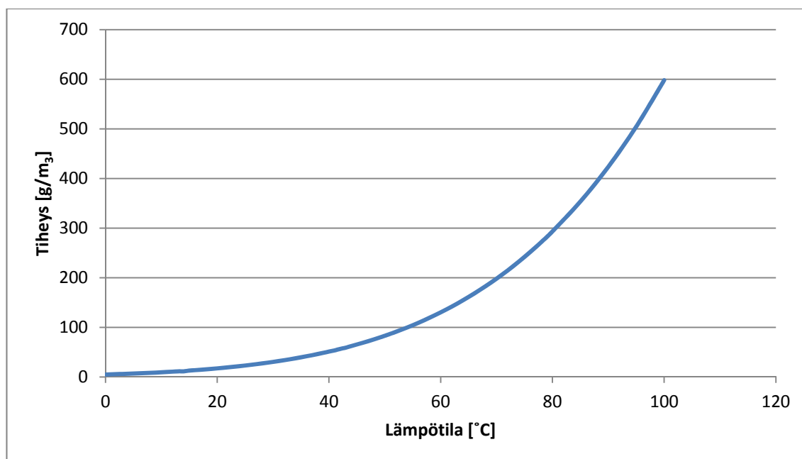
Kuva 5.21. Kylläisen vesihöyryn tiheys lämpötilan funktiona.
