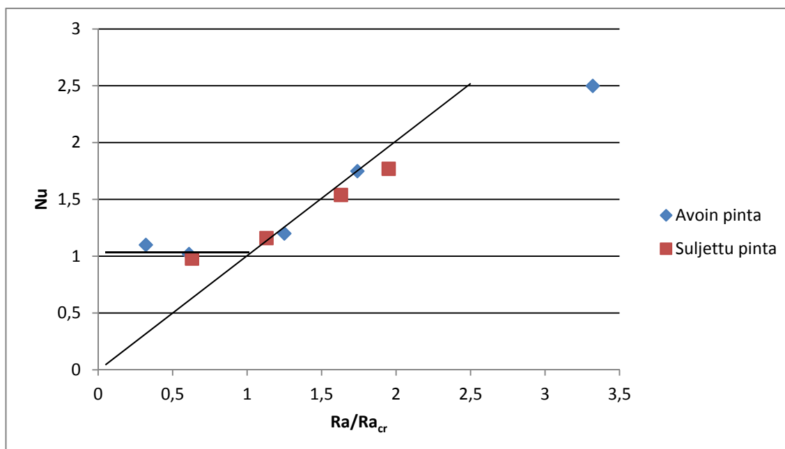
Kuva 3.1. Johansenin testitulokset. Mitattu Nusseltin luku piirrettynä suhteessa laskettuun Ra/Ra_{cr} . Avoimella pinnalla Ra_{cr} on 27 ja suljetulla 41.
