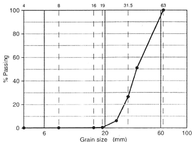
Kuva 3.3. Goering et al. käyttämän materiaalin rakeisuuskäyrä. Vertailun vuoksi Suomessa käytössä olevan raideseppelin minimirakeisuus on 31,5 mm. (Goering et al. 2000)
