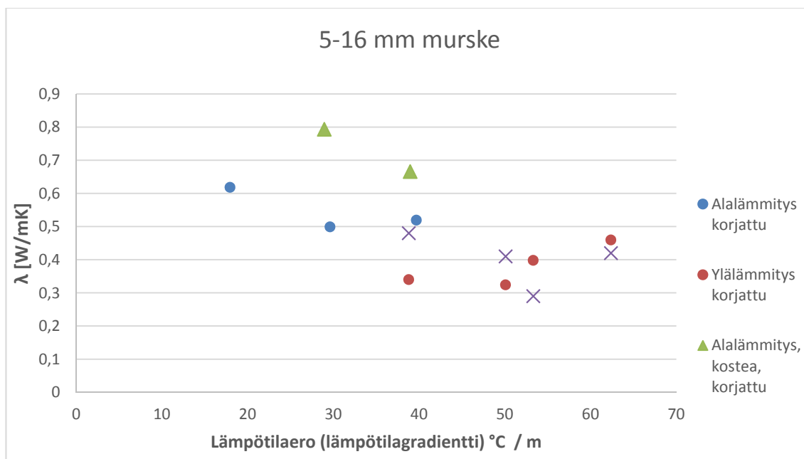
Kuva 5.19. Korjatut lämmönjohtavuudet 5/16 mm kalliomurskeelle.
