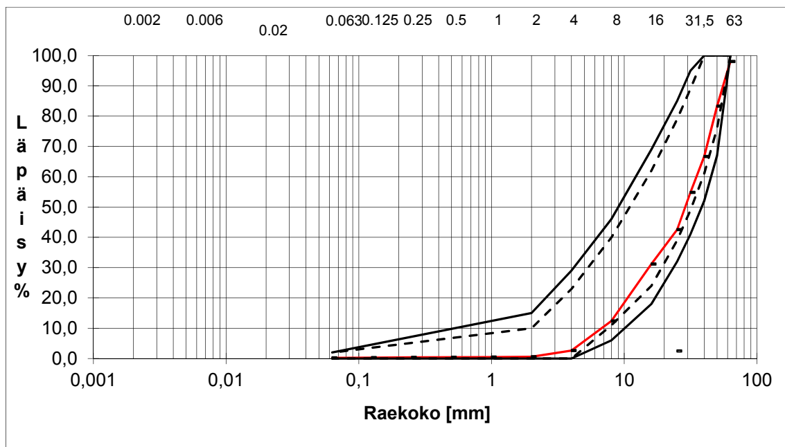
Kuva 4.24. Tutkimusta varten valmistetun eristys-välikerrosmateriaalin raekokojakauma. Kuvassa mustalla piirretyt yhtenäiset viivat ovat yksittäisen rakeisuustuloksen vaihteluvälit. 90 % tuloksista tulee sijaita katkoviivoilla piirretyllä alueella.
