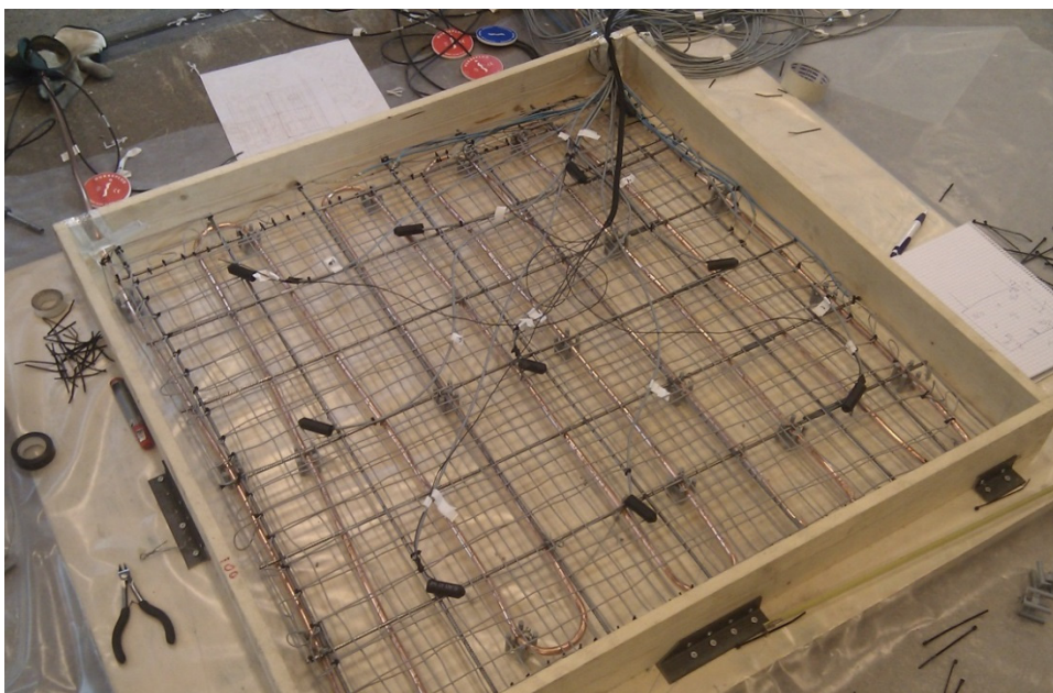
Kuva 4.10. Lämpötila-anturit ennen valua. Kuvassa näkyy 10 kpl LM335 anturia (isot mustat) sekä viisi termoparianturia, jotka ovat samoissa paikoissa. Lämpötila-antureiden alla näkyy harmaa silikonijohdosta tehty lämmitysverkko.
