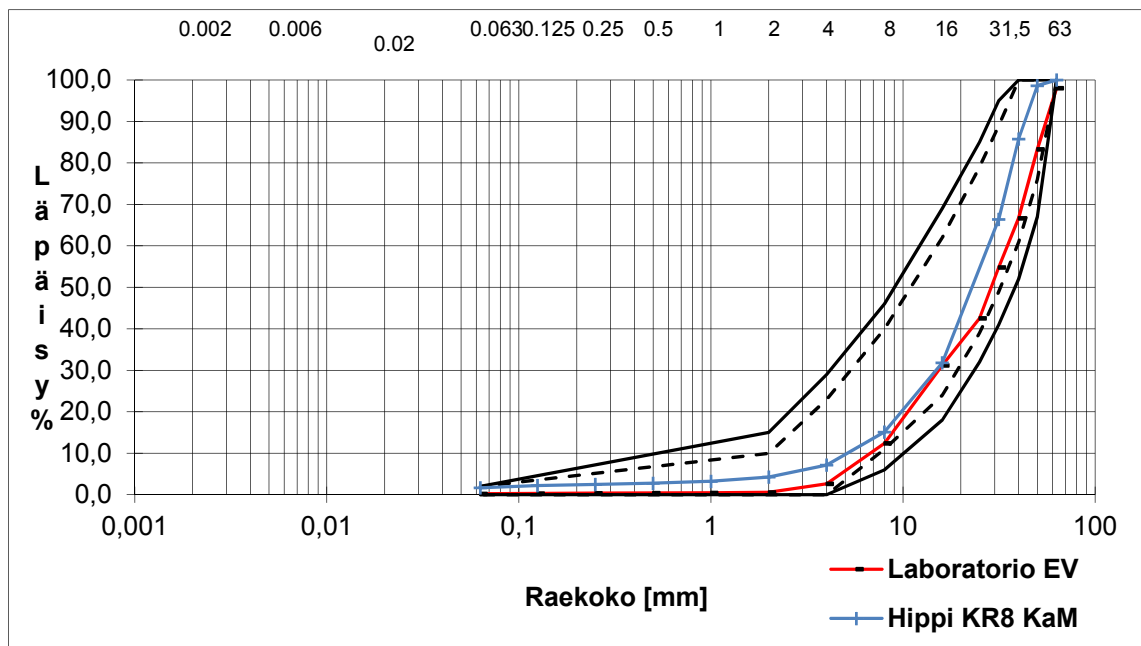
Kuva 6.4. Hipin koekohteessa käytetyn kalliomurskeen rakeisuuskäyrä verrattuna laboratoriotesteissä käytettyyn EV-materiaaliin.
