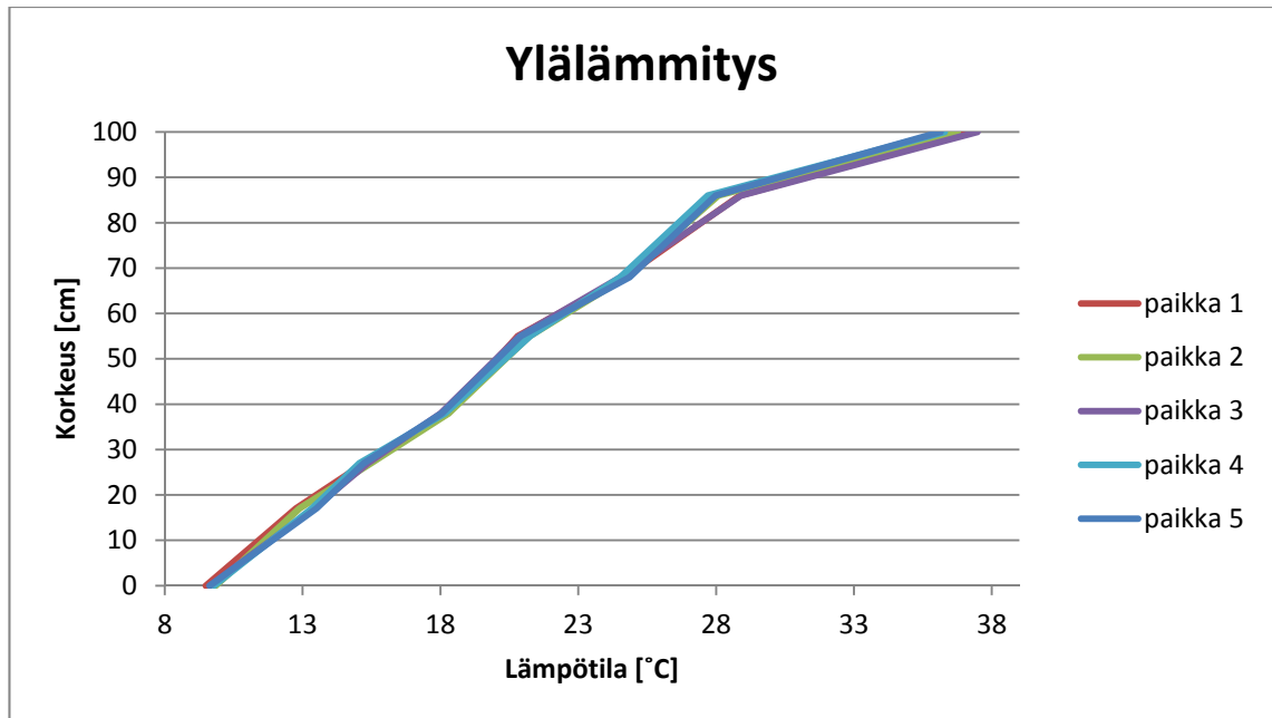
Kuva 5.8. Lämpötilat korkeuden suhteen ylälämmityksellä. Samalla tasolla olevissa lämpötila-antureiden lukemien välillä ei ole havaittavissa merkittäviä eroja. Pienet erot johtunevat anturien sijaintien pienestä heitosta.
