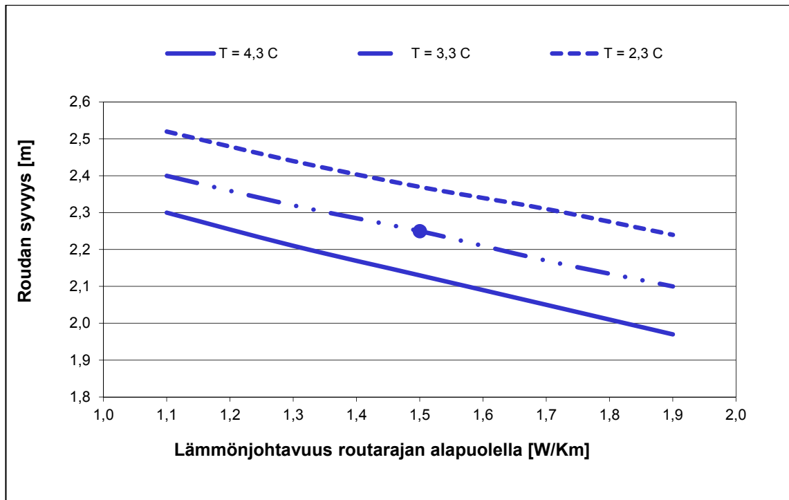
Kuva 2.6. Beskowin menetelmällä tehty roudan syvyyden herkkyydystarkastelu sulan maan lämmönjohtavuudelle ja vuotuisille ilman keskilämpötilalle. Lämpötilagradientti määrätty kaavan G_+ = 0,47 * T_u + 1,4 mukaan. (Nurmikolu & Kolisoja 2002)
