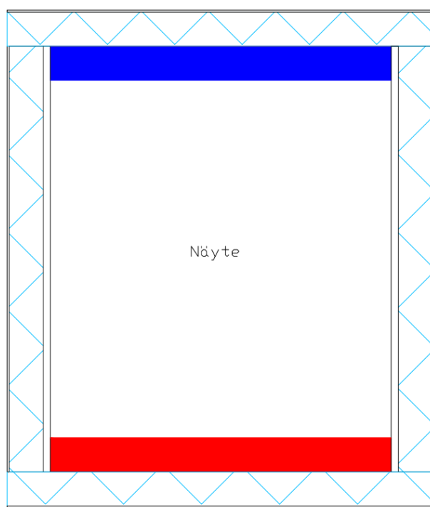
Kuva 4.4. Konvektiolaitteen perusrakenne poikkileikkauksena. Seinärakenne sisältä ulospäin on 28 mm filmivaneri, 100 mm XPS-eriste, 6 mm filmivaneri ja ulkopuolella lisäksi 50x100 mm puut tukemassa rakennetta. Lämmönsiirtolaatat on merkitty kuvaan sinisellä ja punaisella.
