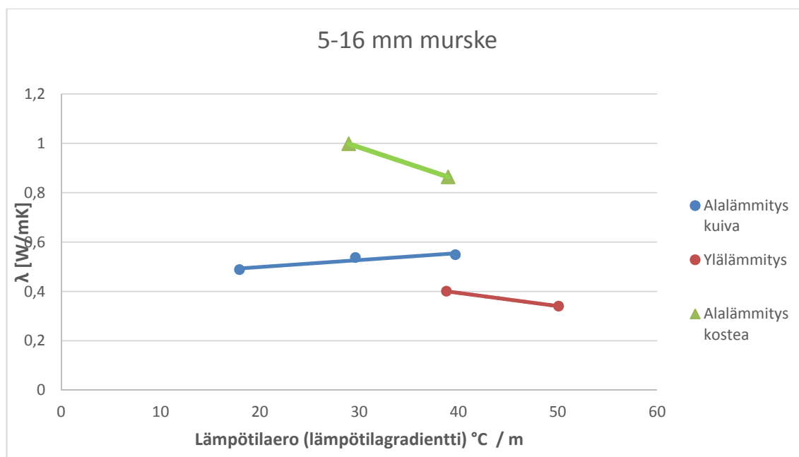
Kuva 5.11. Mitatut lämmönjohtavuudet 5/16 mm kalliomurskeelle
