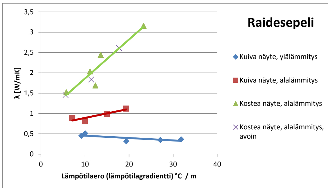
Kuva 5.6. Raideseppelinäytteestä testatut lämmönjohtavuudet lämpötilaeron funktiona 1,0 m korkealla näytteellä.
