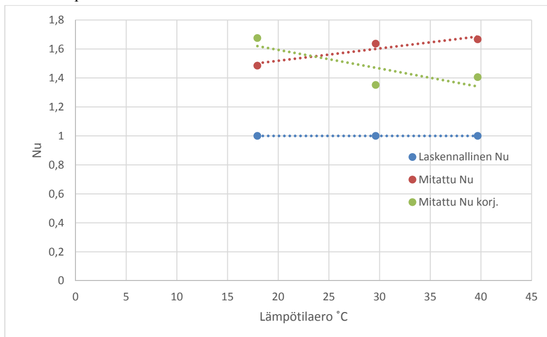
Kuva 5.25. Laskettu ja mitattu Nusseltin luku 5/16 mm kalliomurskeelle. Kuvassa on myös korjatuilla arvoilla laskettu versio. Nusseltin luvun määritelmän takia Nu on aina vähintään yksi.
