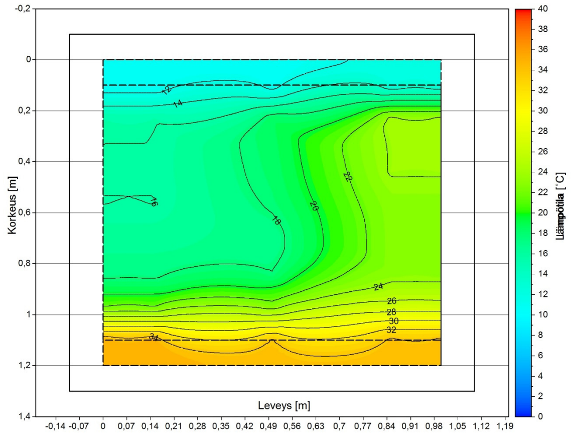
Kuva 5.2. Kostean raidesepelinäytteen isotermit alälämmitystilanteessa. Lämpötilaero on noin 23 °C. Näytteen oikea puoli on selvästi vasenta lämpimämpi.
