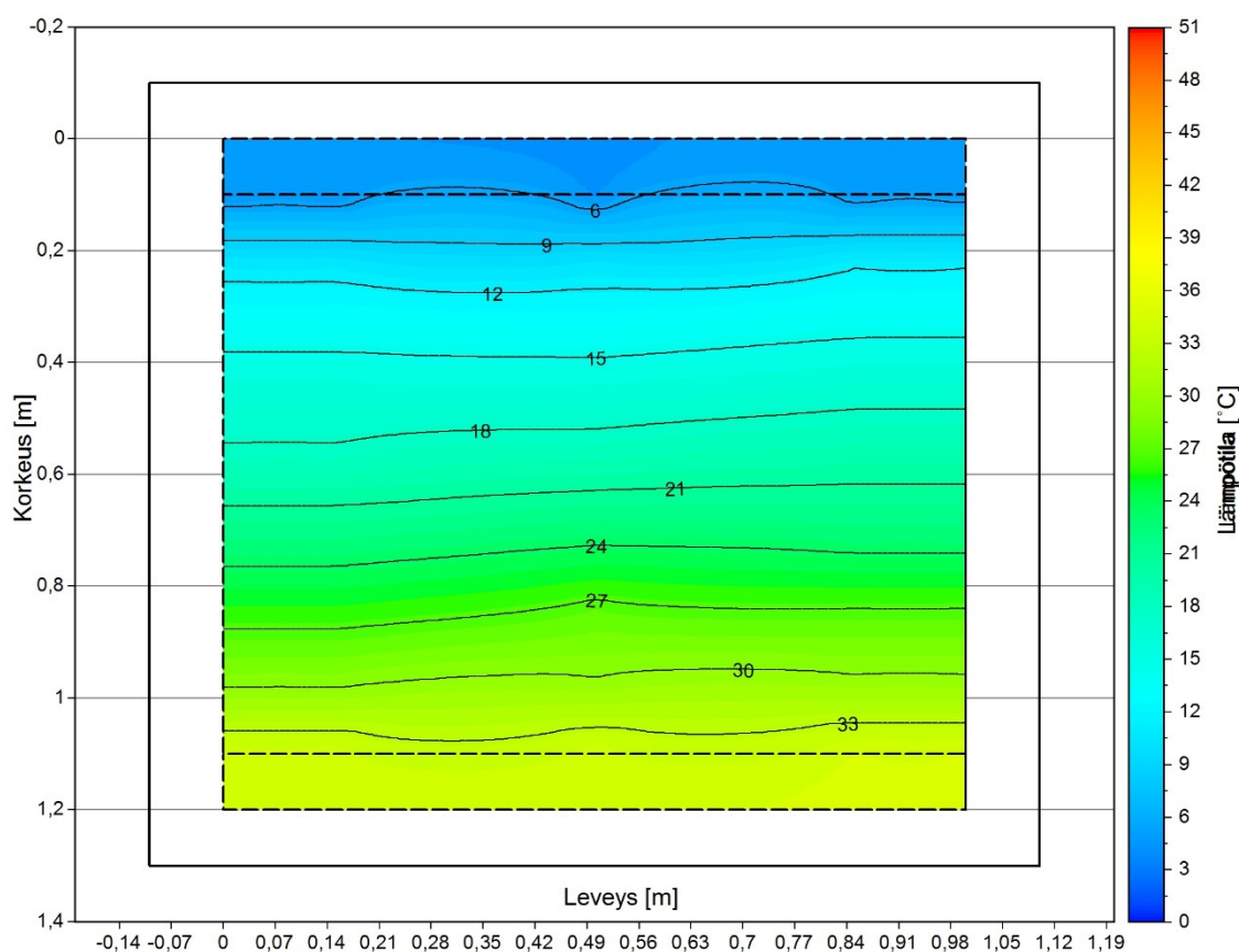
Kuva 5.14. Kuivan EV-materiaalin lämpötilajakaumat alalämmitystilanteessa. Lämpötilaero oli noin 30°C. Isothermit näyttäisivät olevan hieman ylempänä oikeassa reunassa. Tilanne kuitenkin muistuttaa konvektiotilanteen sijaan enemmän johtumistilannetta.
