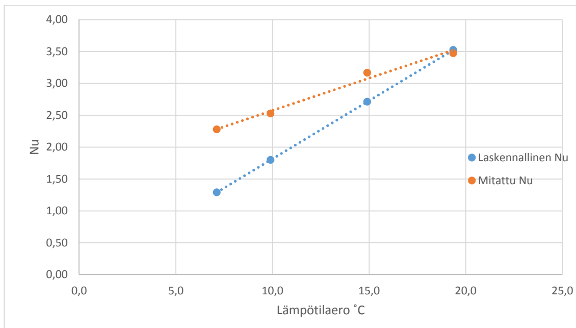
Kuva 5.23. Mitattu ja laskettu Nu raidesevelille käyttäen lämpöhävikkelaskelmalla korjattua lämmönjohtavuutta. Mittaus ja laskennallinen analyysi korreloivat hyvin. Kuvassa on käytetty suoraan mitattua lämmönjohtavuutta 0,36 W/mK.
