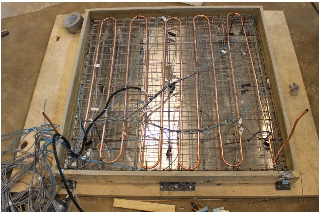
Kuva 4.13. Näytteen päällä oleva lämmönsiirtolaatta. Laatassa olevat rakenteet on katsuttu alalaatan peilikuvana, ja ne ovat näytteen suhteen samoin päin. Ylälaatassa ei ole lämpövuoantureita. Myös johdot ja kupariputket lähtevät ylöspäin, jotta laatta voi vapaasti kellua näytteen päällä.
