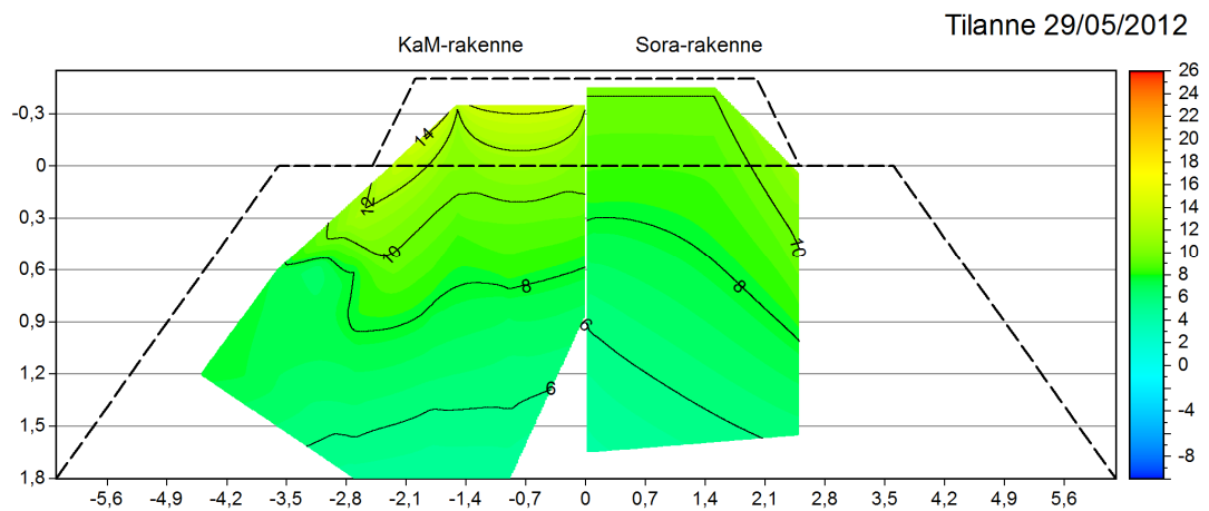
Kuva 6.13. Lämpötilat penkereissä 29.5.2012. Kalliomurskeesta rakennettu ratapenger on lämmennyt myös keväällä 2012 nopeammin verrattuna sorapenkereeseen.
