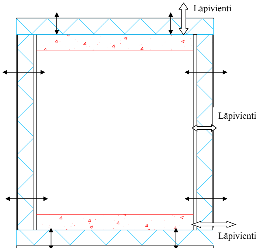
Kuva 4.28. Tutkimuslaitteiston lämpötekninen rakenne poikkileikkauksessa. Ohuet nuolet kuvaavat lämpövuotoja, paksut nuolet ovat läpivientejä, jotka on tiivistetty.
