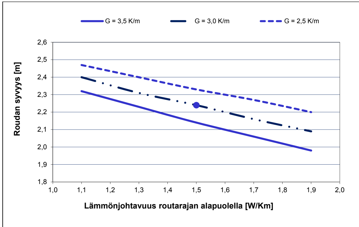
Kuva 2.5. Beskowin menetelmällä tehty roudan syvyyden herkkyydystarkastelu sulan maan lämmönjohtavuudelle ja lämpötilagradientille eristämättömässä rakenteessa. (Nurmi-kolu & Kolisoja 2002)
