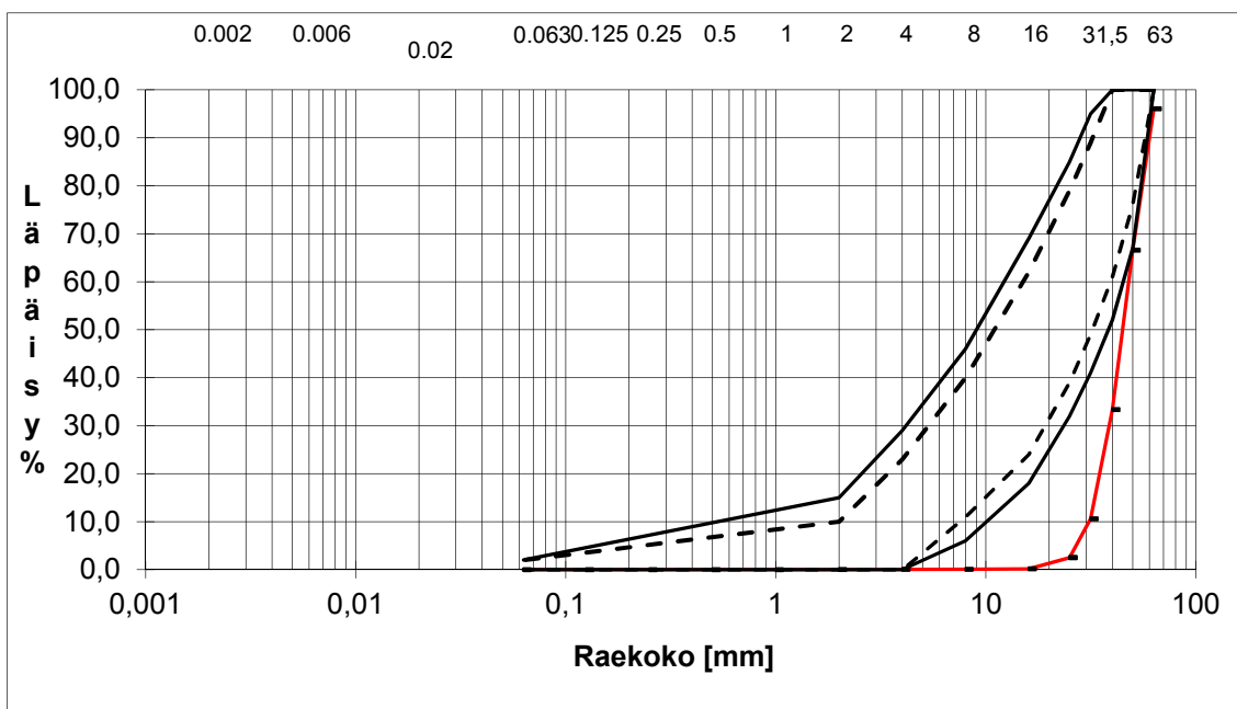
Kuva 4.20. Testattavan raideseppelin raekokojakauma. Kuvassa mustalla piirretyt yhtenäiset viivat ovat yksittäisen rakeisuustuloksen vaihteluvälit EV-materiaalille. 90 % tuloksista tulee sijaita katkoviivoilla piirretyn alueen sisäpuolella.
