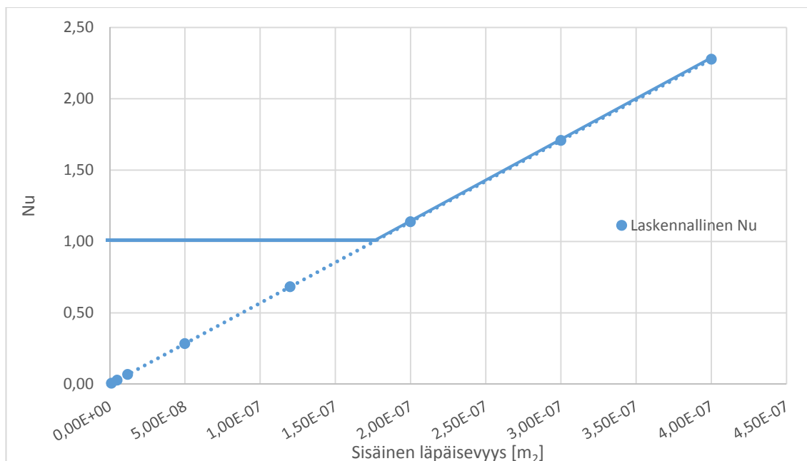
Kuva 5.28. EV-materiaalille laskettu Nusseltin luku kokeen parametreilla sisäisen läpäisevyyden mukaan. Nusseltin luku ei teorian mukaan voi olla alle yhden, joten alle yhden oleva osuus on merkitty katkoviivalla.
