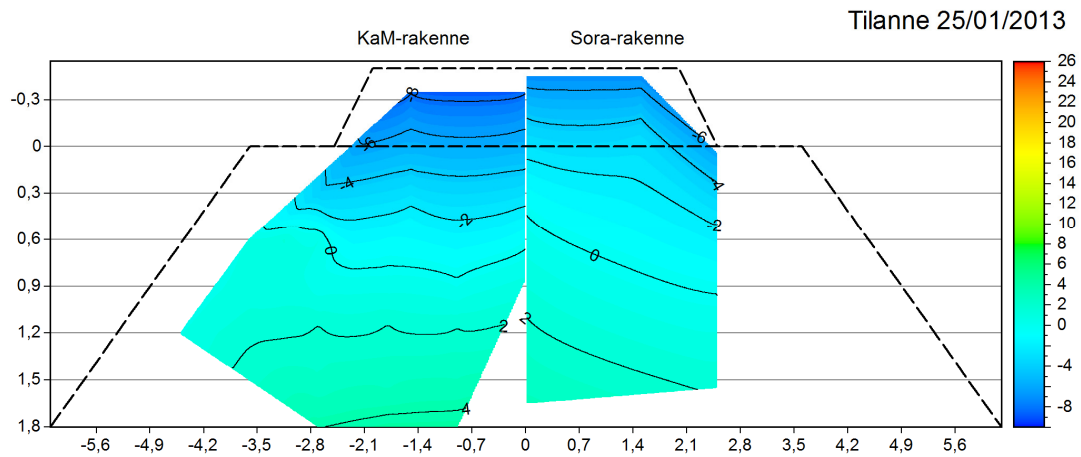
Kuva 6.15. Lämpötilat penkereissä 25.1.2013. Kalliomurskerakenne on alaosistaan sorarakennetta lämpimämpi mutta yläosistaan kylmempi.
