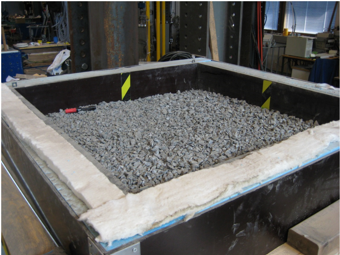
Kuva 4.23. Testattava 5/16 mm kalliomurske konvektiolaitteessa.
