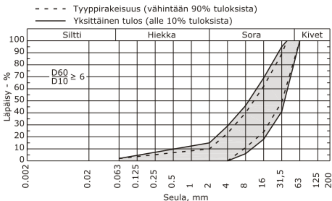
Kuva 2.10. Radan eristyskerroksen ja välikerroksen rakeisuusvaatimukset kalliomurskekerrokselle. (InfraRYL 2012)
