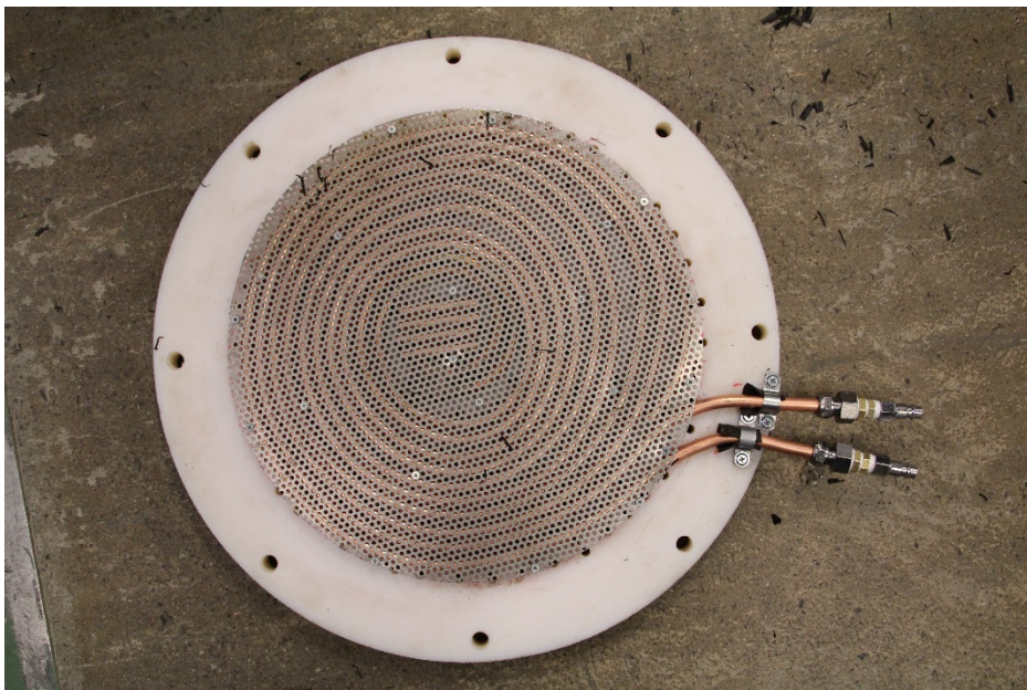
Kuva 4.3. Konvektiolaitteen prototyypin kuparikierukkälämmönvaihdin. Näytteen päällä ja alla oli samantyyppiset lämmönvaihtimet, joiden läpi ilma pääsi virtaamaan. Ylempi lämmönvaihdin sopi putken sisään.
