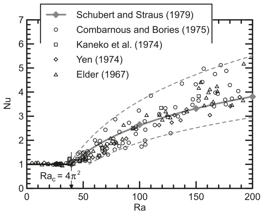
Kuva 3.8. Nusseltin luku suhteessa Rayleighin lukuun eri tutkimuksissa. Tulokset ovat kokeellisia & analyttisiä tuloksia huokoiselle materiaalille suljetussa neliön muotoisessa laatikossa. (Côté et al. 2011)
