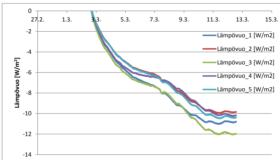
Kuva 5.7. Nopeustestin tulokset. Lämpövuoto kasvaa melko nopeasti sen jälkeen, kun jäähdytys on aloitettu. Ajankohtana 4.3. kuvassa lämpövuomittureiden välillä alkaa näkyä eroa, joka viittaa konvektion alkamiseen.
