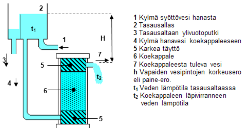
Kuva 4.26. Vedenläpäisevyyskokeen mittauslaitteiston periaate. (kuva MPR:n raportointipohjasta)
