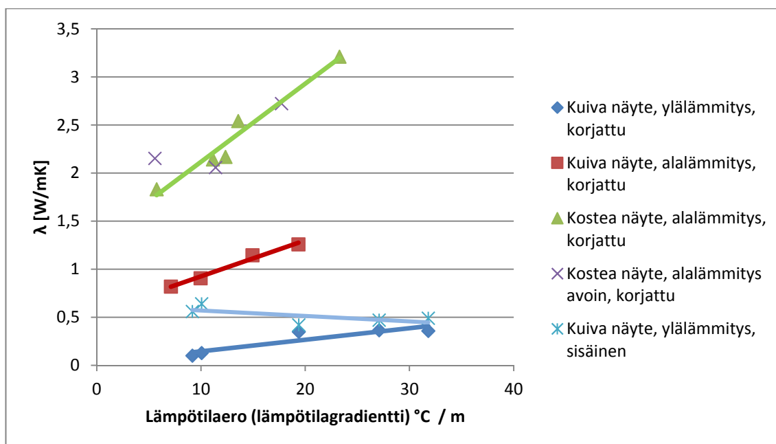
Kuva 5.18. Raidesepelinäytteen lämpöhävikkilaskelmalla korjatut lämmönjohtavuudet lämpötilaeron funktiona 1,0 m korkealla näytteellä.
