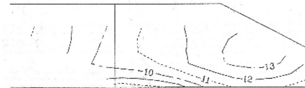
Kuva 3.7. Goeringin testipenkereen isotermit helmikuussa 1994. Kuvasta on havaittavissa, että isotermit poikkeavat selvästi lineaarisesta tilanteesta, jossa lämpöä siirtyy vain johtamalla. Penkereen päällä on ollut 100 mm jääkerros ja luiskissa tiivistämätön lumi. (Goering 1998)
