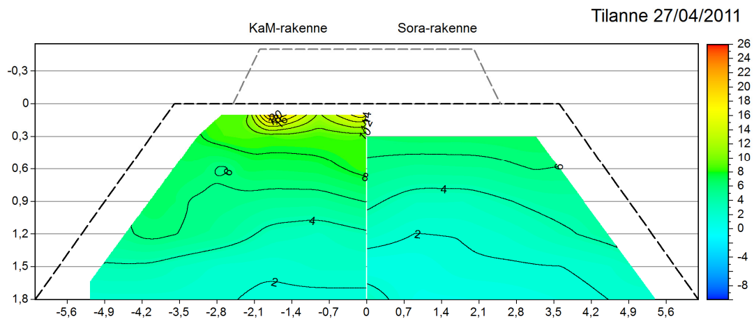
Kuva 6.10. Lämpötilat penkereissä 27.4.2011. Kalliomurskepengen on lämmennyt yläosasta, reunoilta ja myös sisäosiltaan nopeammin kuin sorarakenteinen ratapenger.
