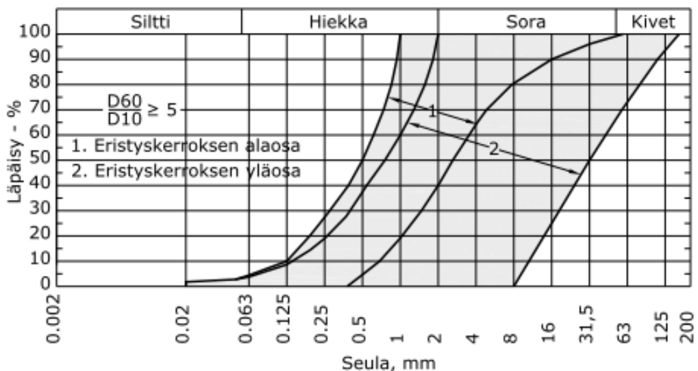
Kuva 2.9. Radan eristyskerroksen materiaalivaatimukset, kuva InfraRYL-julkaisusta. Käyrän tulee noudattaa rajakäyrien muotoa. (InfraRYL 2012)
