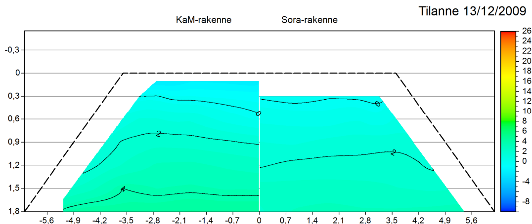
Kuva 6.11. Lämpötilat penkereissä 13.12.2009. Kalliomurskeesta rakennettu ratapenger on syvältä lämpimämpi kuin sorapenger.
