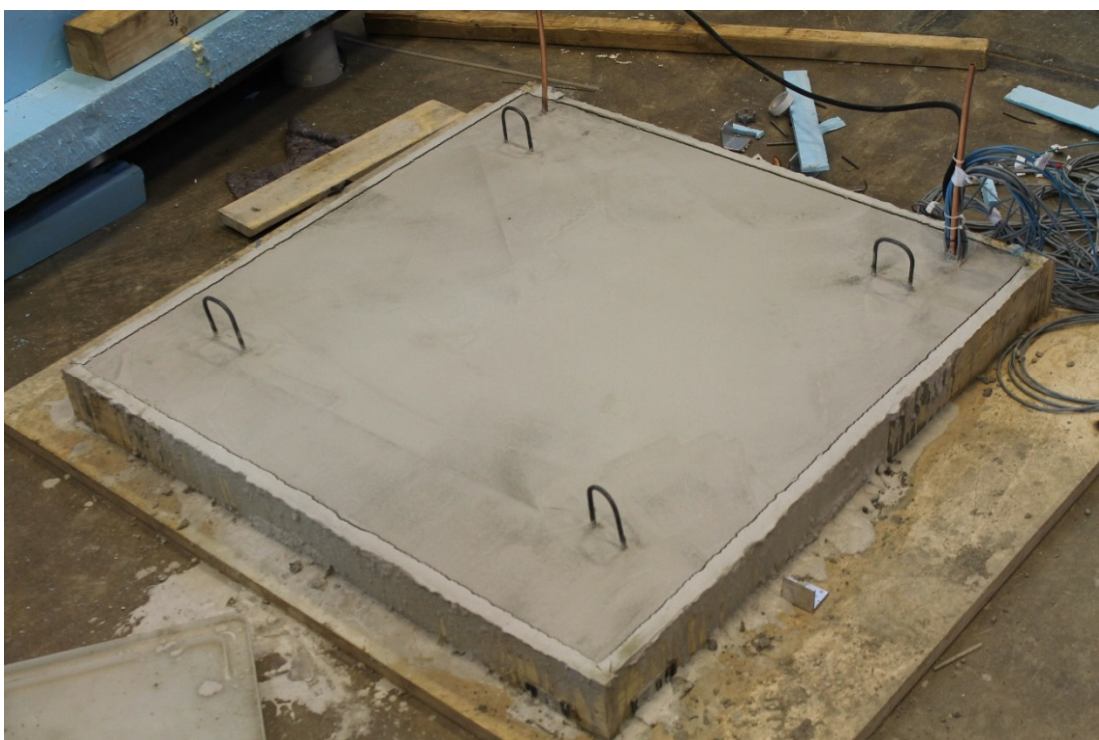
Kuva 4.14. Ylälaatta valun jälkeen. Laatan pintaan on asennettu nostokoukut, jotta painavaa laattaa voidaan siirtää siltanosturilla.
