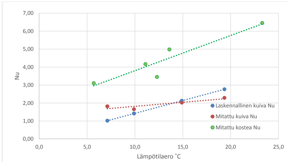
Kuva 5.24. Nusseltin luvut lämpötilaeron suhteen raidesepeissä. Kuvaan on piirretty myös kostean tilanteen testin tulokset. Nusseltin luvut on laskettu käyttäen sisäistä lämmönjohtavuutta 0,49 \text{ W/mK} .
