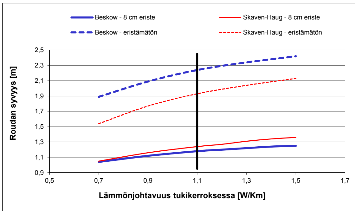
Kuva 2.3. Roudansyvyyslaskelmien herkkyytarkastelu tukikerroksen lämmönjohtavuuden mukaan. (Nurmikolu & Kolisoja 2002)
