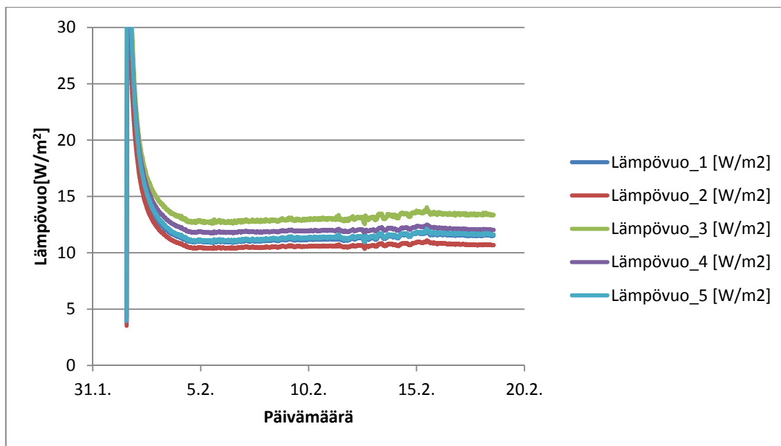
Kuva 4.31. Näytteen lämpövirtaustilan tasaantuminen. Lämpövuotantureiden lukemista on nähtävissä, ettei lämpövuoto muutu enää merkittävästi. Tasaantuneesta tilanteesta on otettu viimeisen 8 tunnin keskiarvo, jonka perusteella tulokset on laskettu. Esimerkkikuva on peräisin raidesepelille tehdystä ylälämmityskokeesta, jossa lämpötilaero oli n. 32 C.
