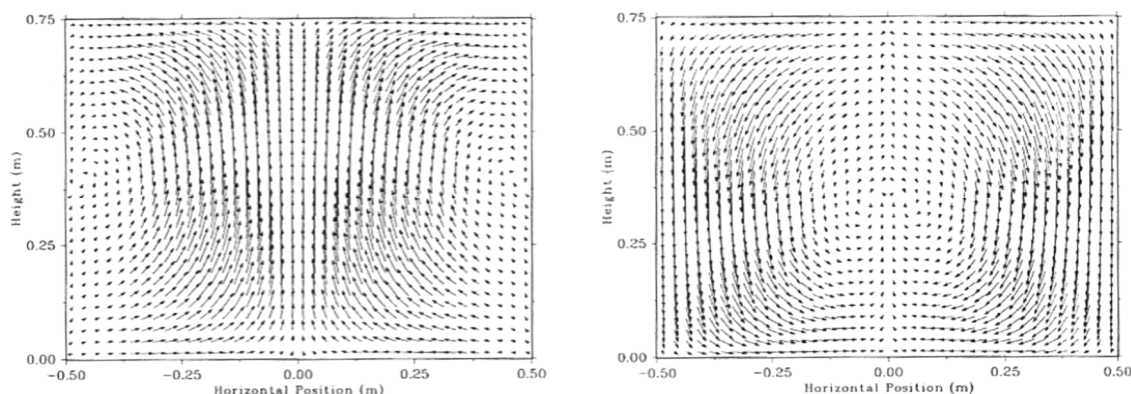
Kuva 3.5. Goering et al. tutkimusryhmän mallinnus ilman kulkemisesta konvektiotilanteessa. Vasemmanpuoleinen kuva on näytteen keskilinjalta ja oikeanpuoleinen reunalta. (Goering et al. 2000)
