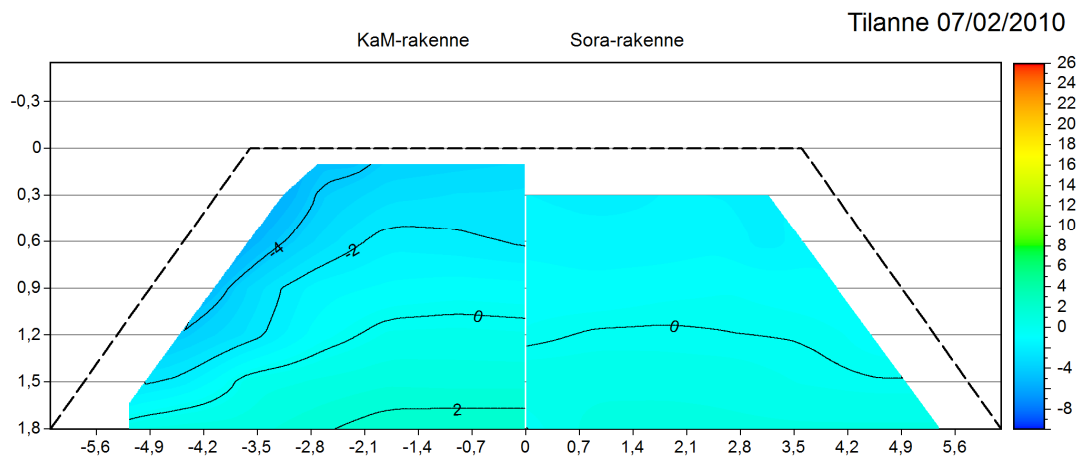
Kuva 6.9. Lämpötilat penkereissä 7.2.2010. Kalliomurskepenkereen reunan lämpötilat poikkeavat selkeästi sorarakenteesta. Sorarakenne on kokonaisuudessaan melko tasalämpöinen verrattuna kalliomurskerakenteeseen.
