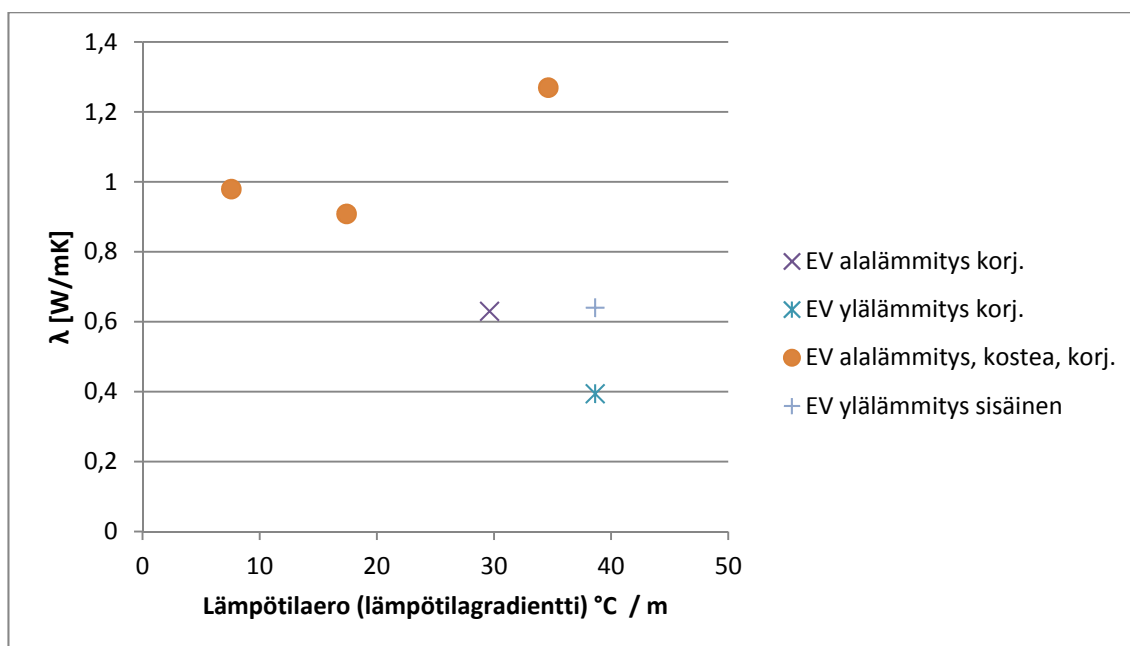
Kuva 5.20. EV-materiaalille lämpöhävikkilaskelman avulla korjatut tulokset sekä näytteen sisäinen lämmönjohtavuus.
