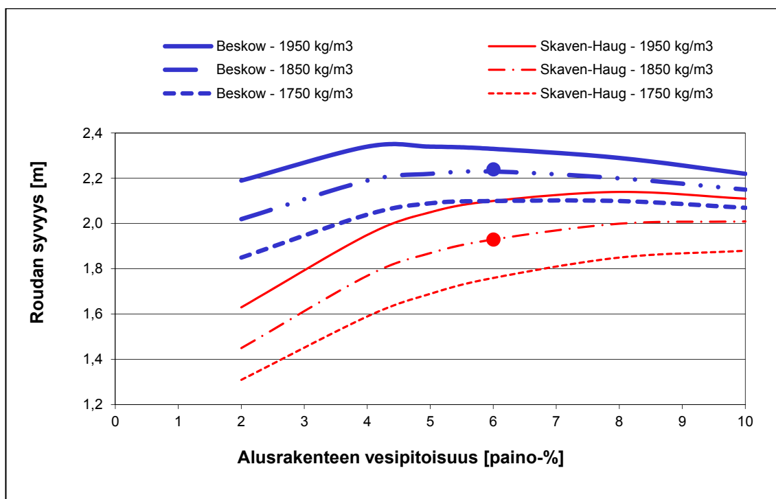
Kuva 2.4. Roudansyvyyslaskelmien herkkyys eristämättömässä rakenteessa alusrakenteen vesipitoisuudelle ja kuivairtitiheydelle. Laskelmissa on oletettu, että lämmönjohtavuus määräytyy vesipitoisuuden ja kuivatiheyden perusteella Kerstenin yhtälöiden mukaisesti. (Nurmikolu & Kolisoja 2002)
