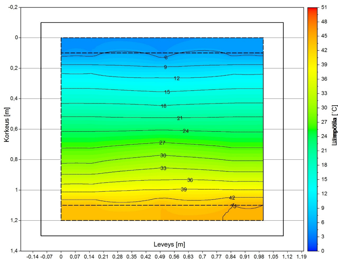
Kuva 5.10. 5/16 mm kalliomurskeen lämpötilajakauma ja isotermit 40^{\circ}\text{C} lämpötilaerolla alalämmitystilanteessa. Isotermeissä on havaittavissa pientä taivutusta keskellä, mutta tilanne muistuttaa kuitenkin johtumistilannetta.
