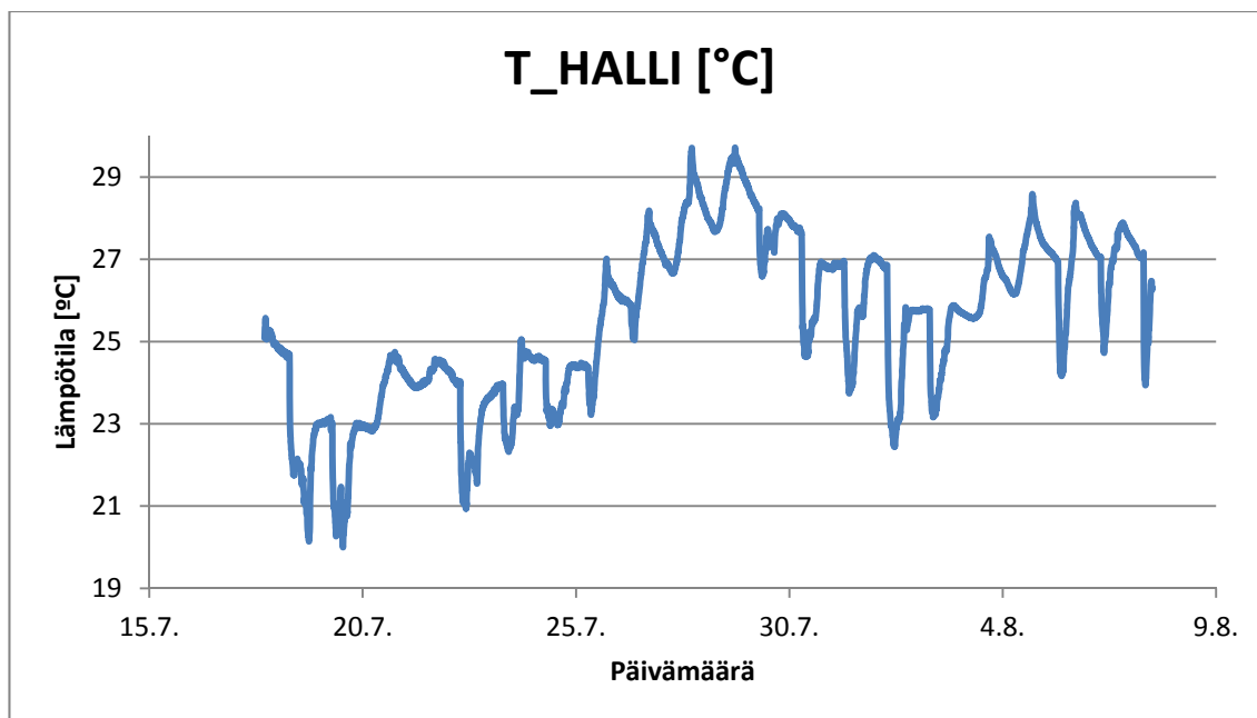
Kuva 4.30. Esimerkki tilanteesta, jossa lämpövuotoa on vaikea laskea.
