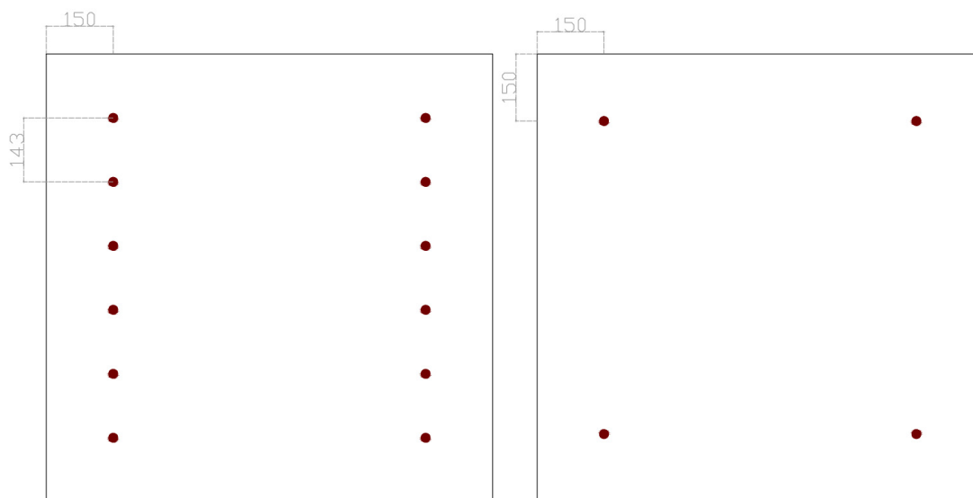
Kuva 4.29. Näytteen reunoilla olevat lämpötila-anturit. Vasen kuva on poikkileikkaus sivultapäin. Oikeanpuoleinen kuva on antureiden sijainti ylhäältä päin katsottuna. Antureita on sijoitettu kuuteen eri kerrokseen tasavälein 150 mm päähän reunoista.
