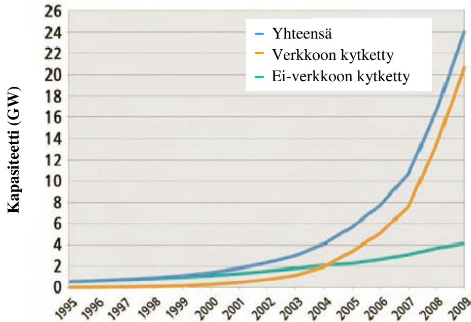
Kuva 4.1. Aurinkosähkön tuotantokapasiteetin kasvu vuodesta 1995 vuoteen 2009. [REN10]
