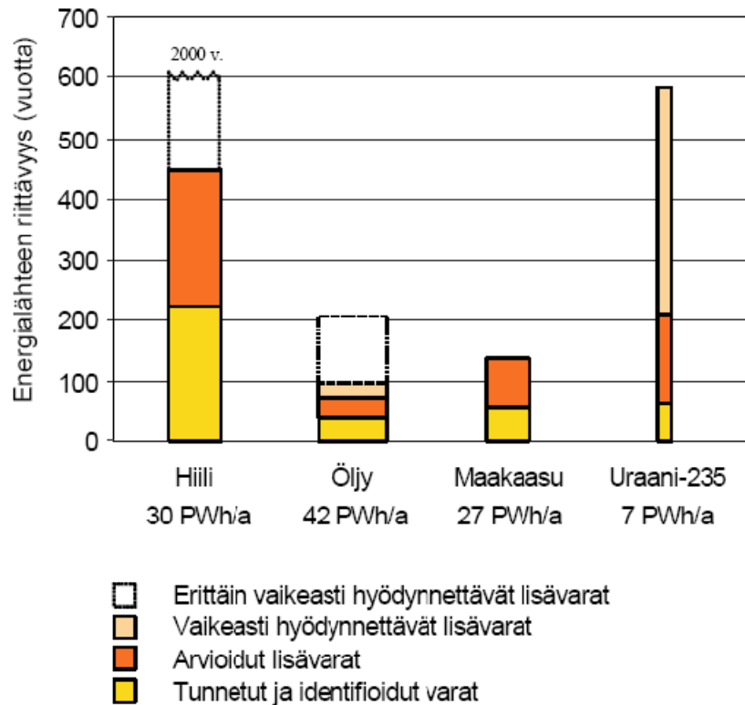
Kuva 2.3. Tunnettujen ja arvioitujen fossiilisten polttoainevarojen riittävyys vuoden 2003 kulutuksella. Hiili sisältää kivihiilen, ruskohiilen ja bitumihien varat. [Ber06]
