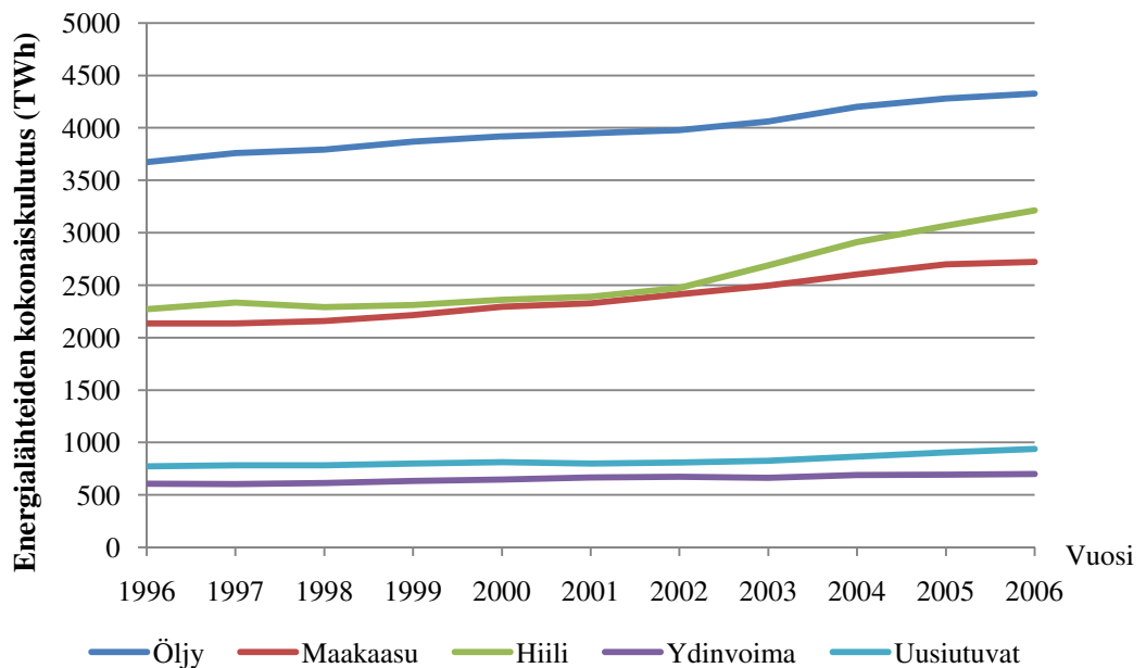
Kuva 2.2. Maailman primäärienergiälähteiden kokonaiskulutuksen kehitys vuodesta 1996 vuoteen 2006. [EIA08b]
