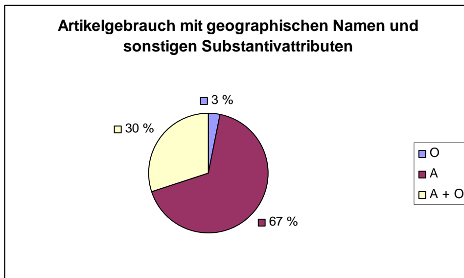
Abb. 4 Artikelgebrauch mit geographischen Namen und sonstigen Substantivattributen
