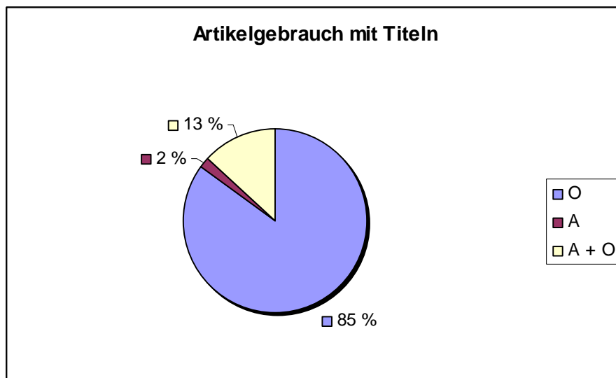
Abb. 1 Artikelgebrauch mit Titeln
