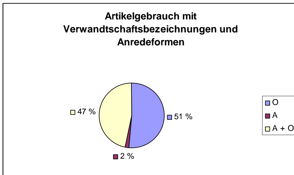
Abb. 3 Artikelgebrauch mit Verwandtschaftsbezeichnungen und Anredeformen
