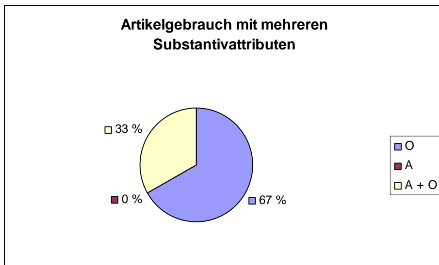
Abb. 5 Artikelgebrauch mit mehreren Substantivattributen
