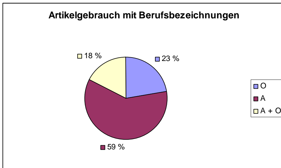
Abb. 2 Artikelgebrauch mit Berufsbezeichnungen
