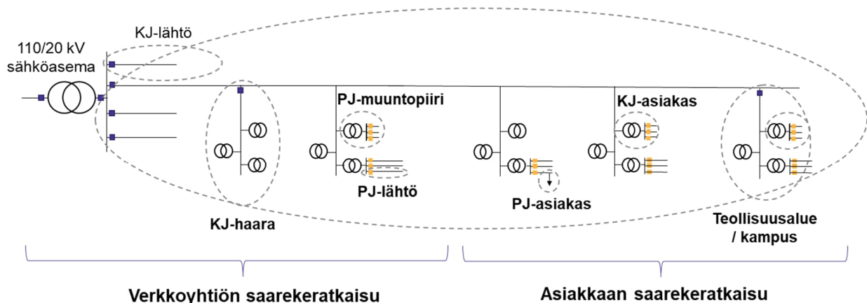
Kuva 2. Saarekeratkaisuvaihtoehtoja
