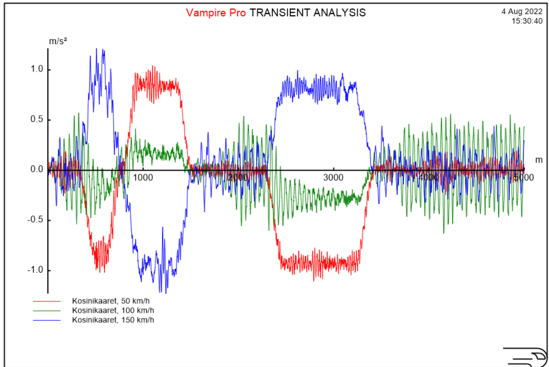
Kuva 26. Poikittaiskiihtyvyyden kuvaajat kosinikaarin lasketusta ratamallista.
