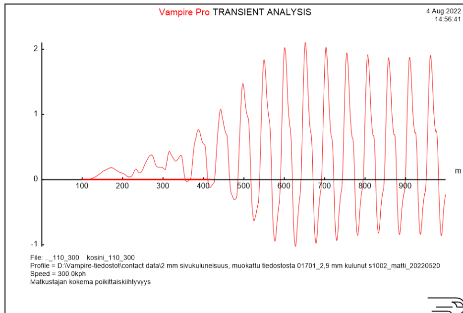
Kuva 37. Poikittaiskiihtyvyys kosinikaaren muotoisessa siirtymäkaaressa nopeudella 300 km/h ja 110 mm kallistuksella. 315 m pitkä siirtymäkaaren osuus esitetty punaisella janalla.
