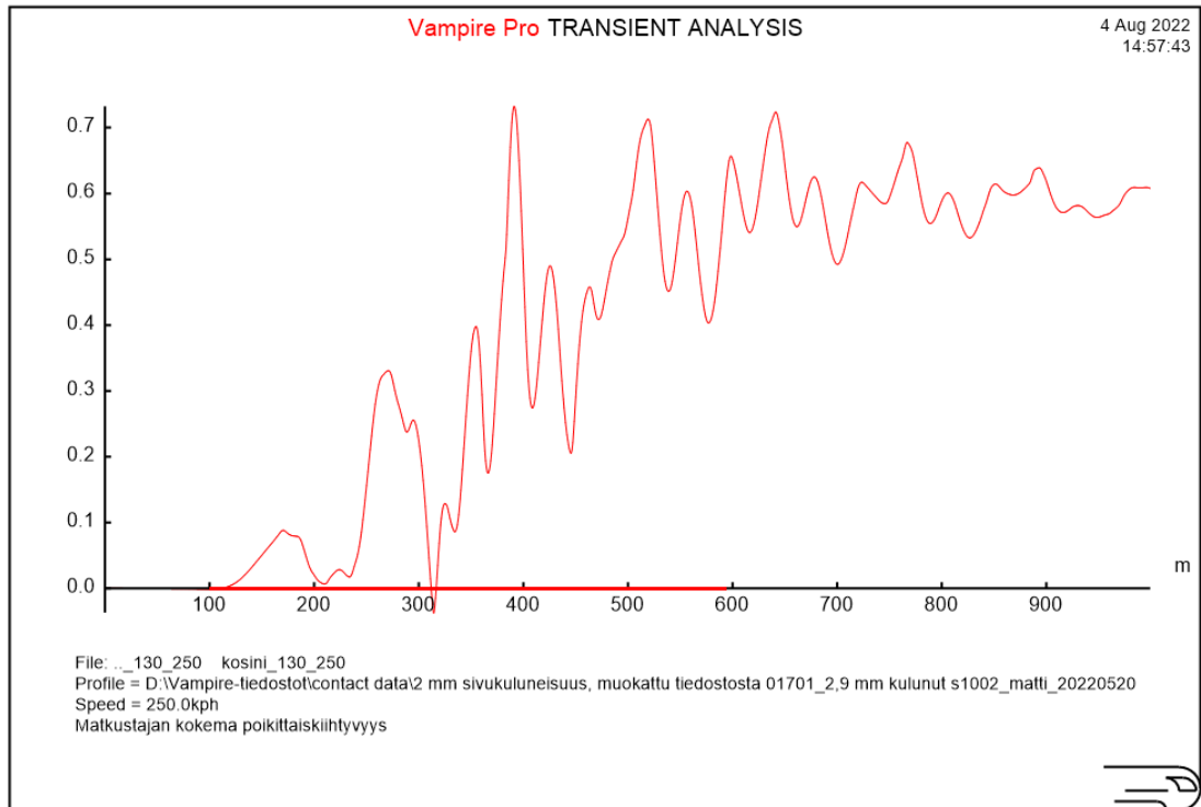
Kuva 38. Poikittaiskiihtyvyys kosinikaaren muotoisessa siirtymäkaarella nopeudella 250 km/h ja 130 mm kallistuksella. 490 m pitkä siirtymäkaaren osuus esitetty punaisella janalla.
