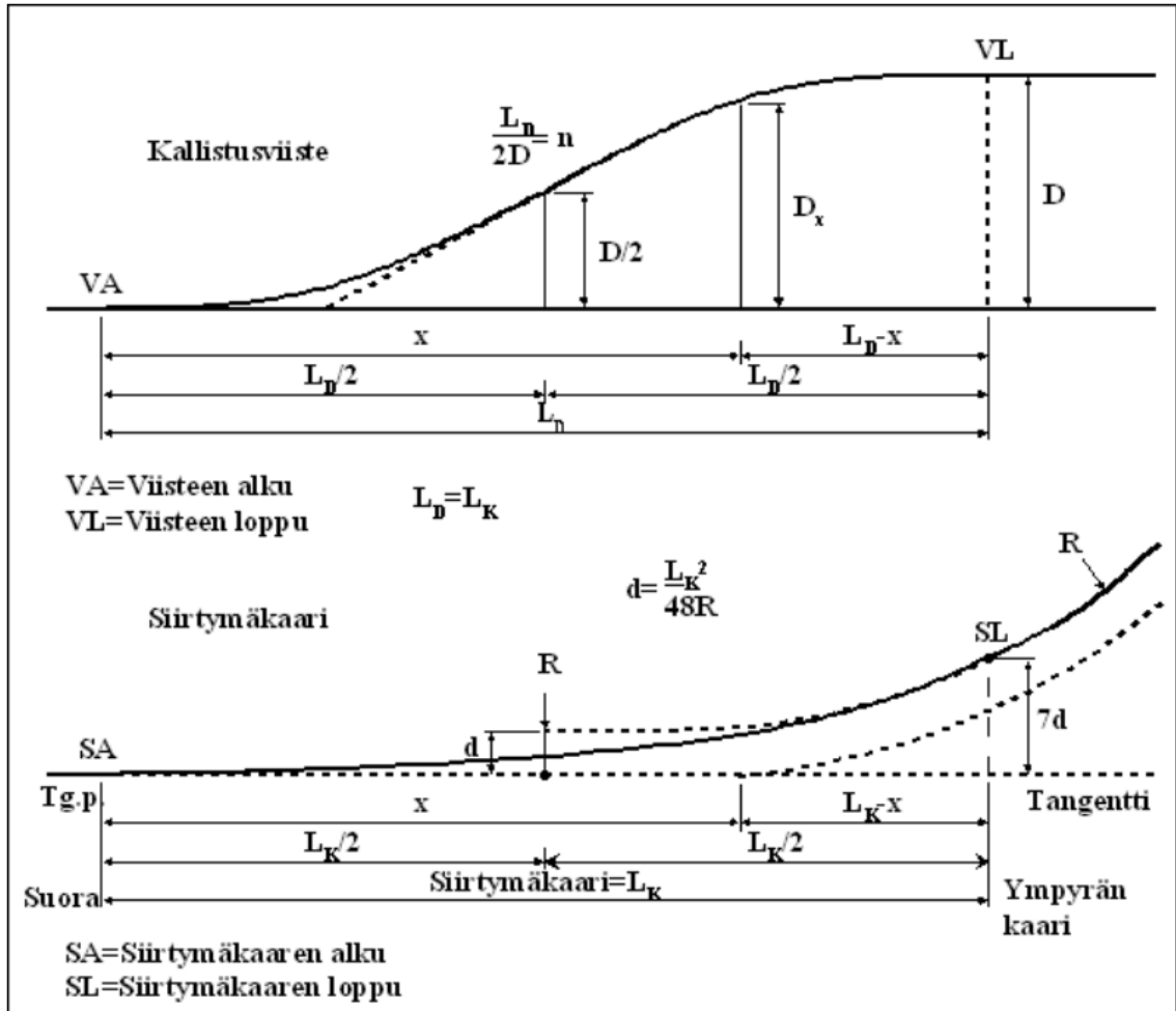
Kuva 9. Helmertin siirtymäkaareissa käytettävä S-kallistusviiste ja sitä vastaava siirtymäkaaren kuvaaja. (Taimela, 2011)
