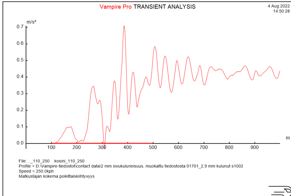
Kuva 36. Poikittaiskiihtyvyys kosinikaaren muotoisessa siirtymäkaaressa nopeudella 250 km/h ja 110 mm kallistuksella. 490 m pitkä siirtymäkaaren osuus esitetty punaisella janalla.
