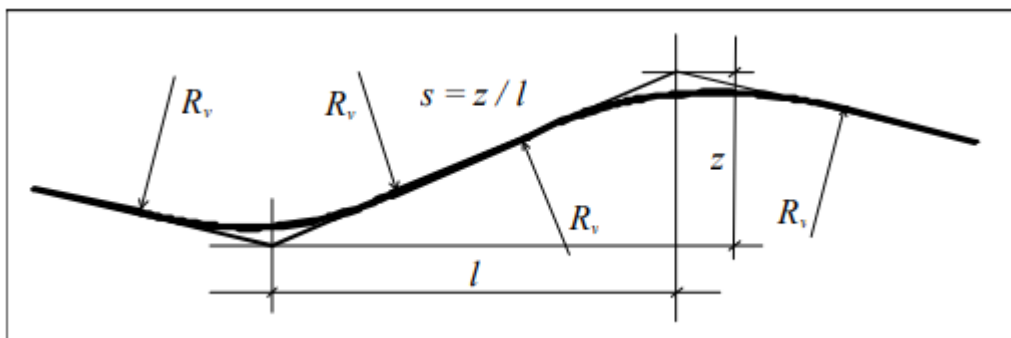
Kuva 5. Kaltevuusjakson pituus, korkeus ja pituuskaltevuus. (Taimela, 2011)
