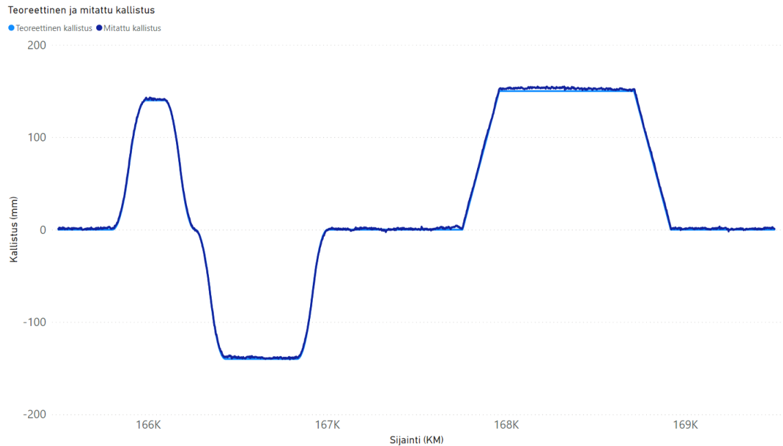
Kuva 15. Laskennallinen ja mitattu kallistus
