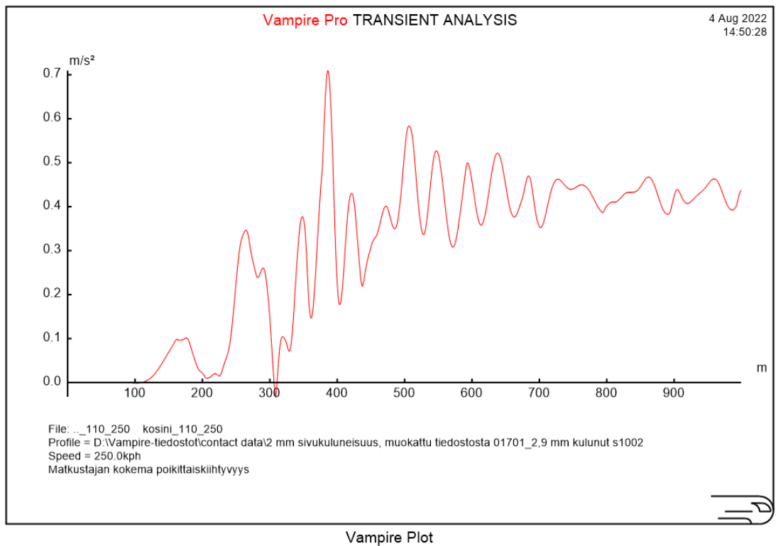
Kuva 39. Poikittaiskiihtyvyys kosinikaaren muotoisessa siirtymäkaarella nopeudella 300 km/h ja 130 mm kallistuksella. 385 m pitkä siirtymäkaaren osuus esitetty punaisella janalla.
