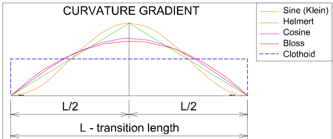
Kuva 7. Eri siirtymäkaarien kaarevuuden muutoksia. (Ciobanu, 2015)
