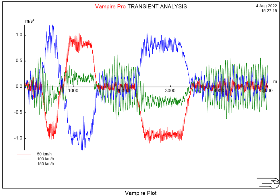
Kuva 24. Poikittaiskiihtyvyyden kuvaajat laskennallisen geometrian avulla luodusta ratamallista. Simlointiajojen nopeudet väreittäin: 50 km/h punaisella, 100 km/h vihreällä ja 150 km/h sinisellä viivalla.
