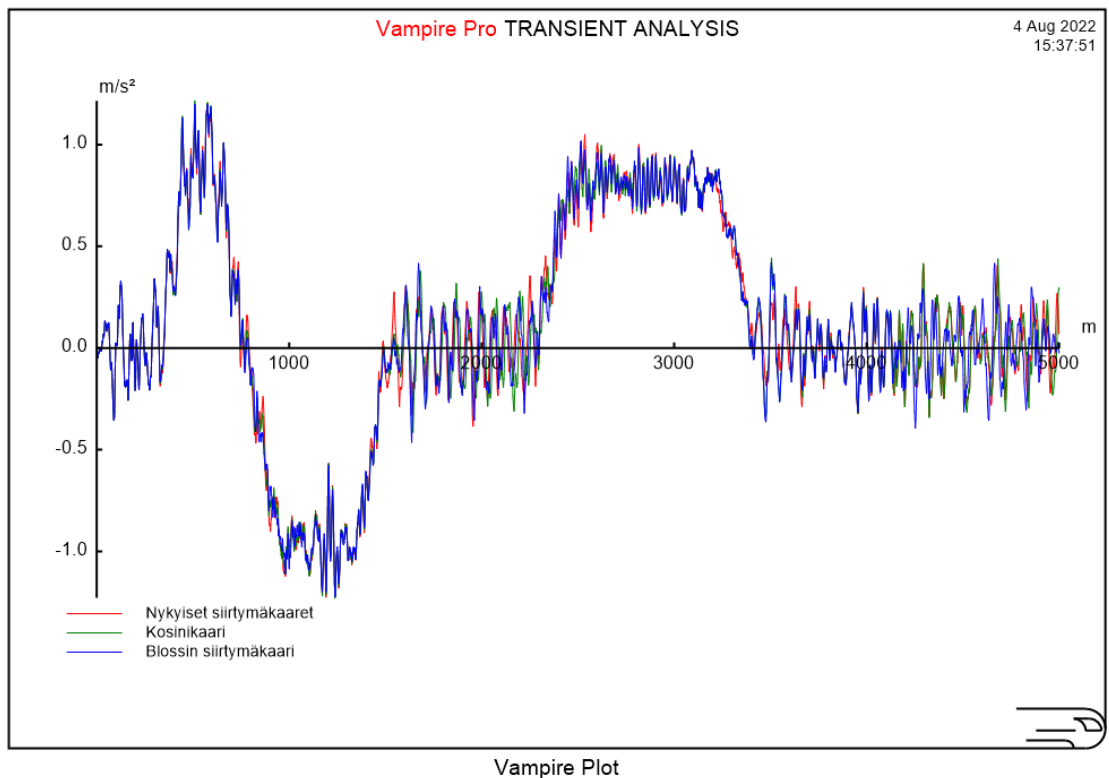
Kuva 27. Poikittaiskiihtyvyyden kuvaajat tutkittavalla rataosalla eri siirtymäkaarin 150 km/h nopeudella.
