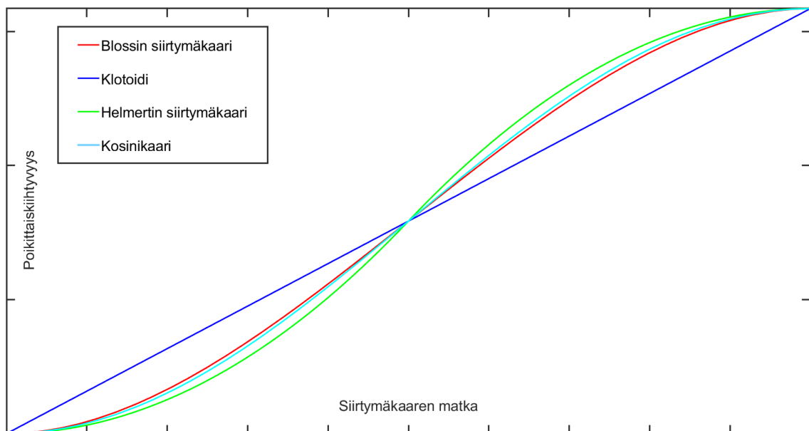
Kuva 11. Poikittaiskiihtyvyyksien kuvaajat eri siirtymäkaarityypeille.
