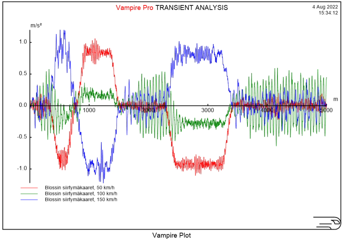
Kuva 25. Poikittaiskiihtyvyyden kuvaajat Blossin siirtymäkaarin lasketusta ratamallista.
