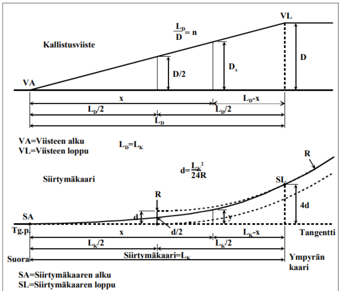
Kuva 3. Siirtymäkaari ja siihen liittyvä suora kallistusviiste. (Taimela, 2011)
