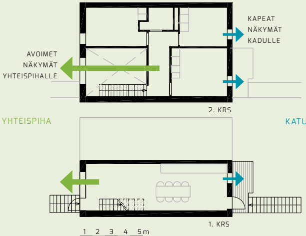
ESIMERKKI KAKSIKERROKSESISTA 97 M 2 ASUNTOPOHJASTA
