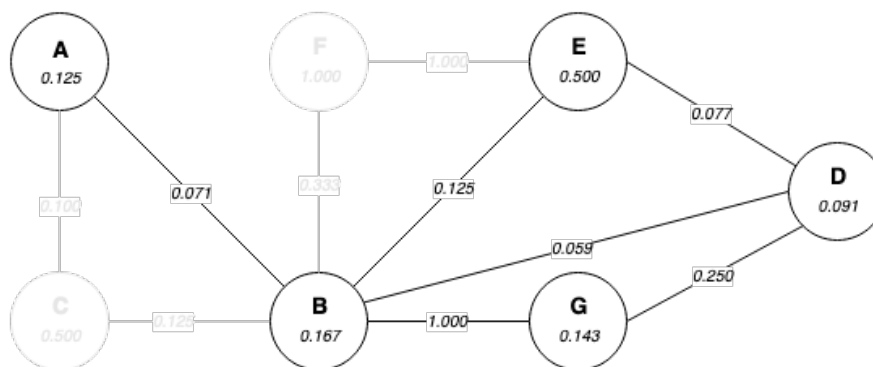
Kuva 5.2. Esimerkin mukainen painotettu verkko leikkauksien jälkeen.
