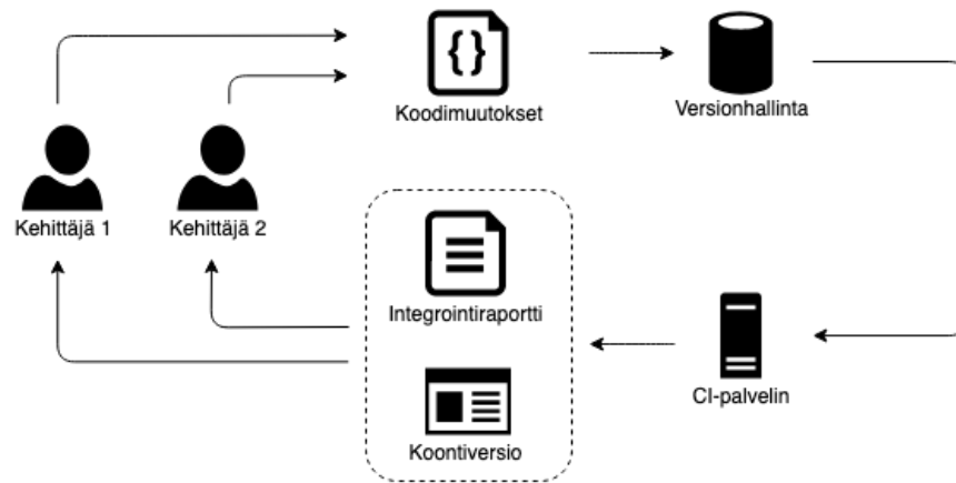
Kuva 3.2. Jatkuvan integroinnin peruseriaate on iteratiivinen.
