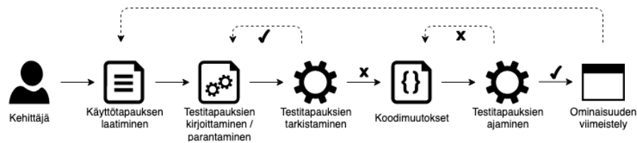
Kuva 4.1. Hyväksymistestausvetoisen kehityksen vaiheet, kuvaa 3.3 mukailleen.
