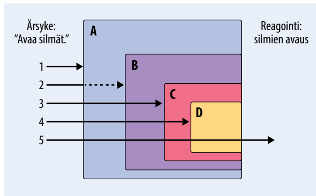
KUVA 1. Tajuiheen reagoitukykyyn vaikuttavat tekijät (4). Aistiärsyke johtaa mielekkääseen vasteeseen vain silloin, kun kaikki tajuihen prosessoinnin osatekijät (A, tajuihen tila; B, tietoisuus ärsykkeestä ja kyky sen ymmärtämiseen) ja toiminnallinen valmius (C, halu ja aikomus reagoida; D, kyky reagoida) toimivat normaalisti. Nuolet kuvaavat ärsyksen prosessointia eri tajunnantiloissa. 1. Mikään ärsyke ei saavuta tajuntaa (esimerkiksi aivokuolema, erittäin syvä anestesia). 2. Unennäkö normaalin unen tai anestesian aikana, jolloin ympäristön ärsykkeet voivat (eivät kuitenkaan välttämättä) vaikuttaa unisälttöön (stimulusinkorporaatio). 3. Haluttomuus reagoida. 4. Kyvyttömyys reagoida (esimerkiksi hereilläolo anestesiassa relaksoituna). 5. Ärsyke johtaa mielekkääseen reagointiin (normaali valveillaolo).
