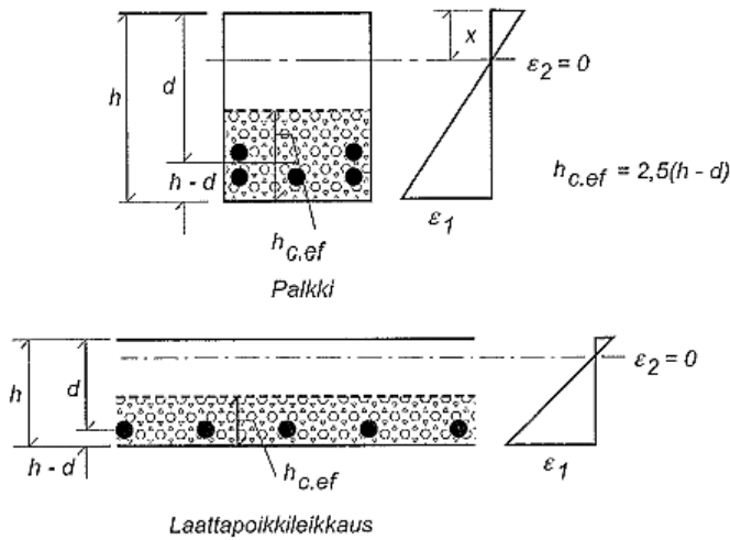
Kuva 18 Teräsiä ympäröivän, vetojännityksen alaisen betonialueen tehollisen pinta- alan korkeus h_{c,eff} , eurokoodin mukaan [46].
