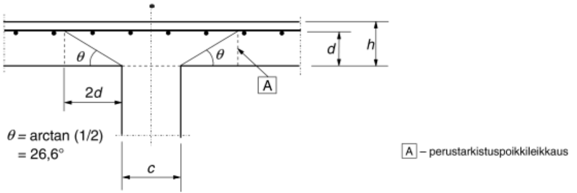
a) Pystyleikkaus
