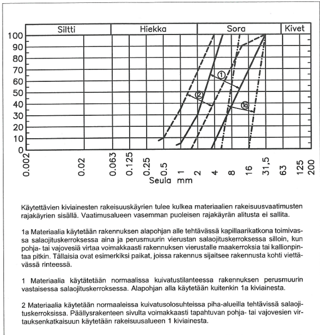
Kuva 3.6. Salaojituskerroksen rakeisuusvaatimukset.
