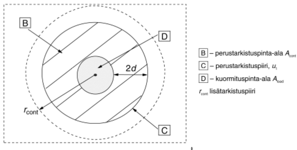
b) Vaakaleikkaus
