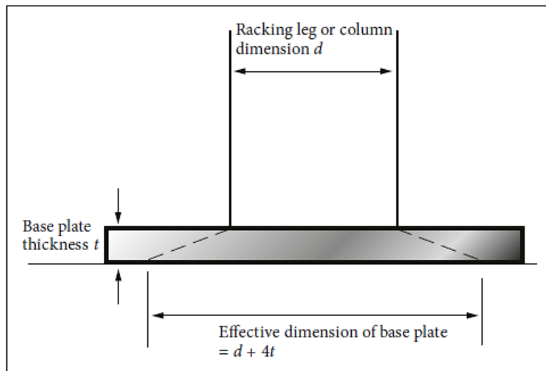
Kuva 8 TR 34:ssä esitetty näkemys pohjalevyn tehollisestä leveydestä [20].
