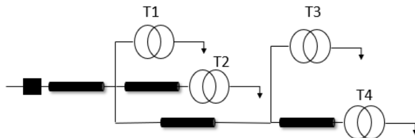
Kuva 33: Yksinkertaistetun verkkomallin varioitavan johtolähdön verkkokaavio.
