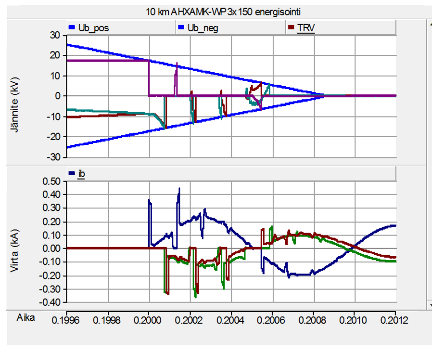
Kuva 24: 10 km AHXAMK-WP 3x150 kaapelin energisoinnin aikaiset esisyytymiset.
