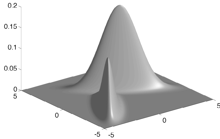
Kuva 2.9: Kaksi erillistä kaksiulotteista normaalijakautunutta komponenttia.
