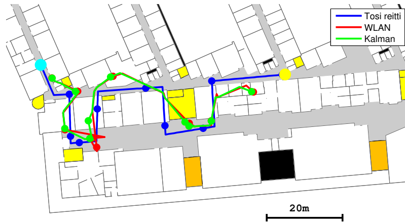
Kuva 5.6: WLAN-paikannuksen ja Kalmanin suodattimen avulla estimoitu testireitti 2.
