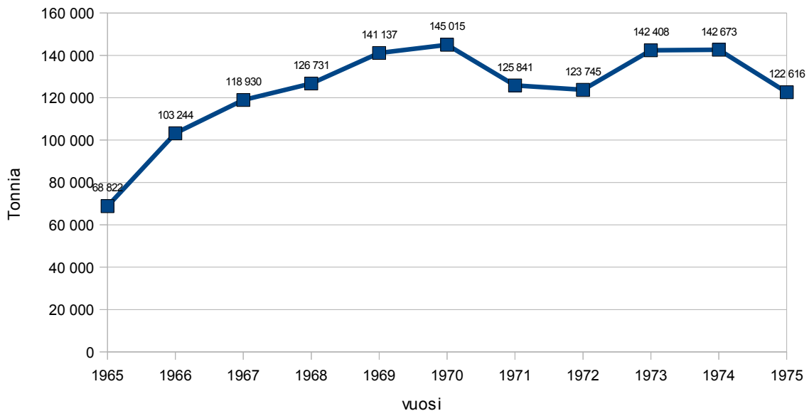
Kaavio 4: Kemijärven selluloosatehtaan myyntituotanto 1965–1975
