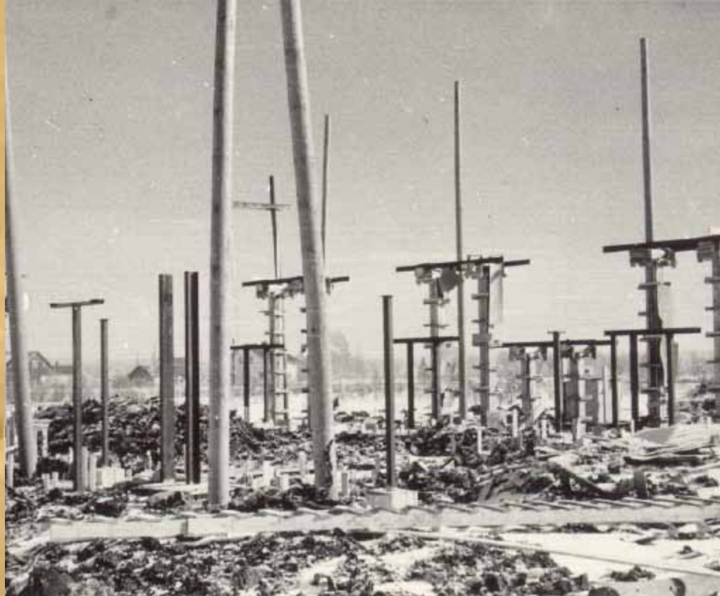
Lapuan Sähkö Oy:n kytkinlaitos keväällä 1955. (EPV)
