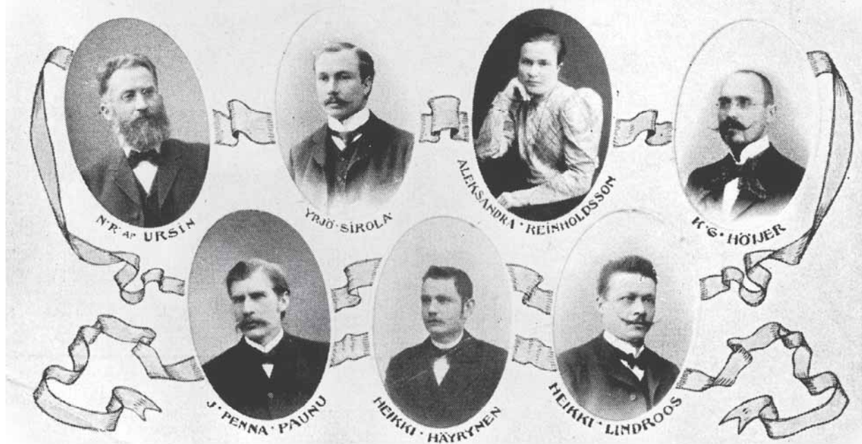
Eduskuntaan 1907 Hämeen läänin pohjoisesta vaalipiiristä valitut sosiaalidemokraatit ryhmäku- vassa. Ylärivissä N. R. af Ursin, Yrjö Sirola ja Aleksandra Reinholdsson, K. G. Höijer. Alarivissä J. Penna Paunu, Heikki Häyrynen ja Heikki Lindroos.
