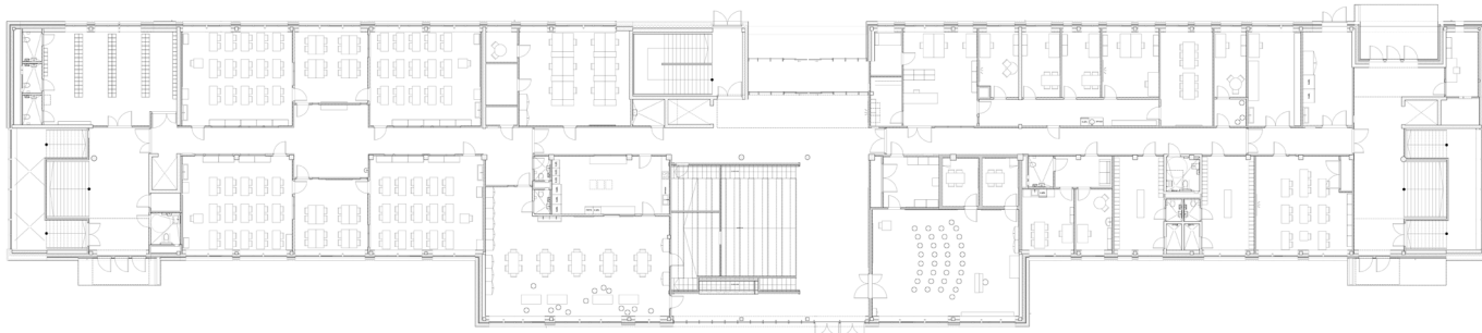
KUVA 3.1.3.b. 1. kerroksen pohjapiirros.
