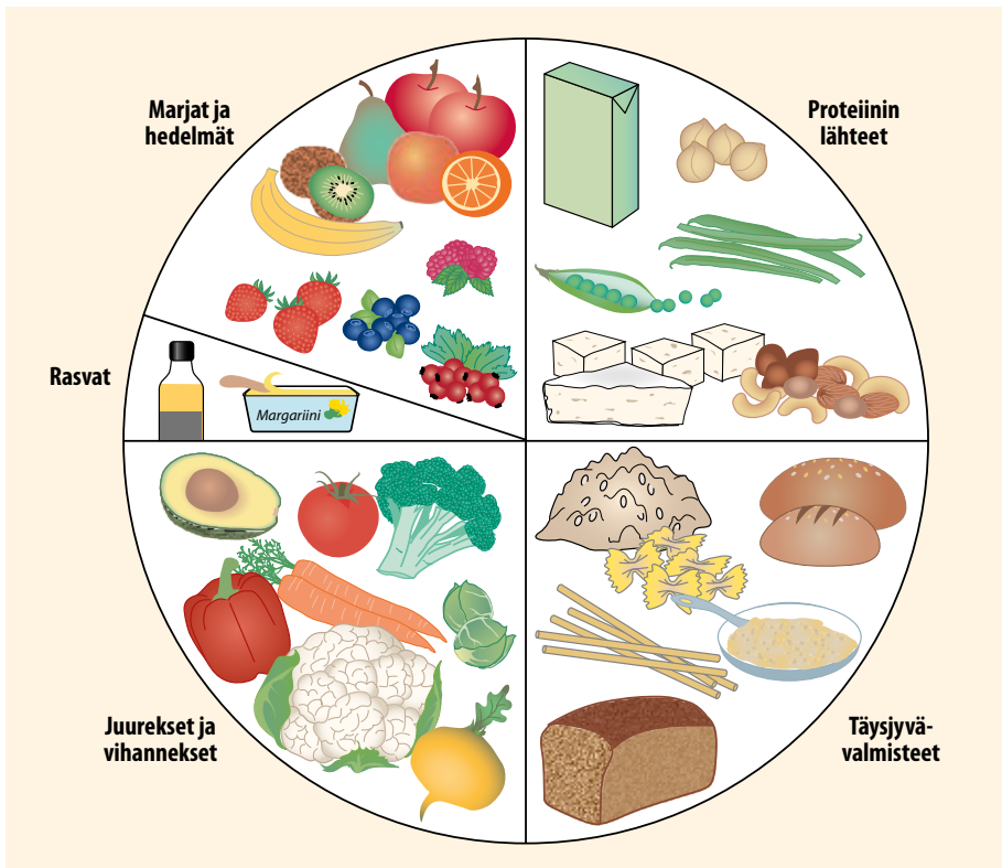
KUVA 2. Vegaanin ruokapyyrä.
