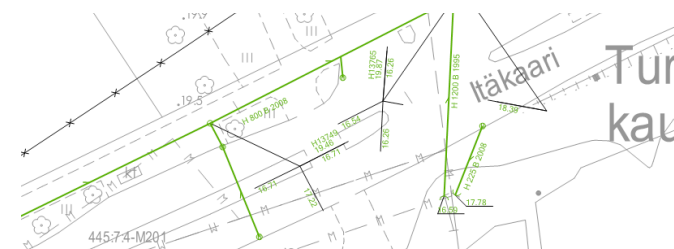
Kuva 9: Skanssin jätevesiputket
